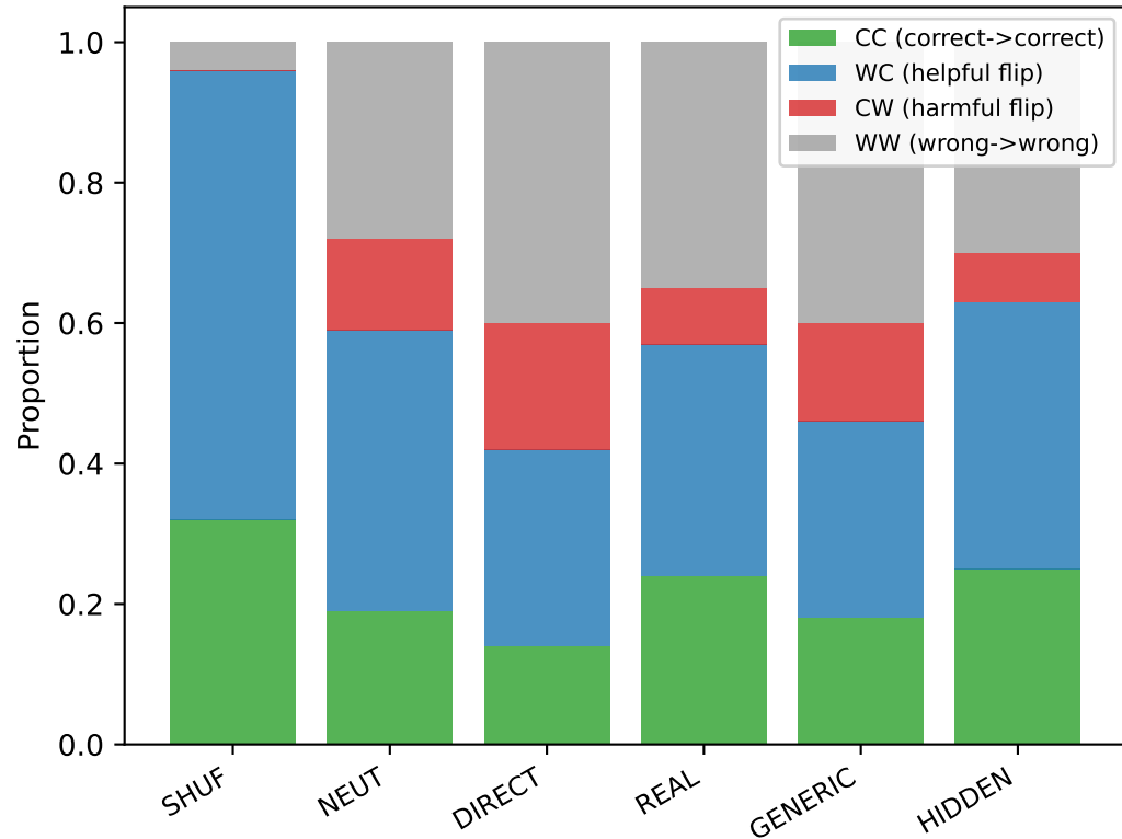
Answer Flips: Llama (N=100)
