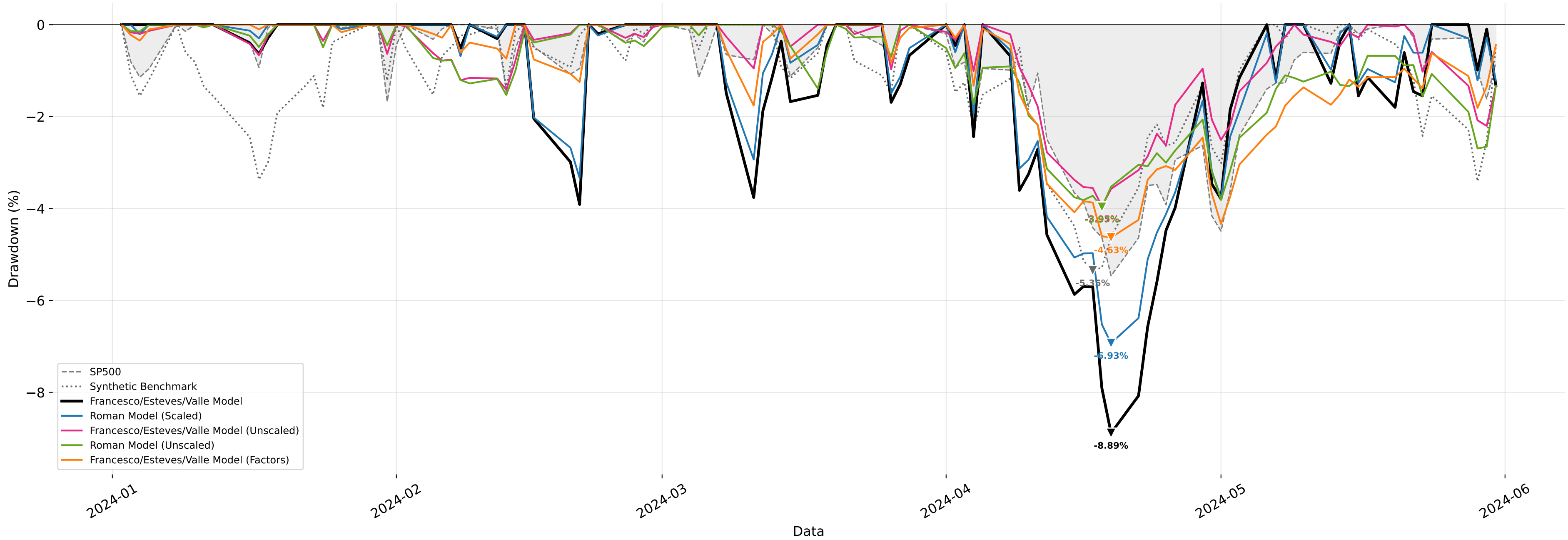
Drawdown — modelos vs Synthetic Benchmark vs SP500 (▼ marca o máximo drawdown de cada série)
