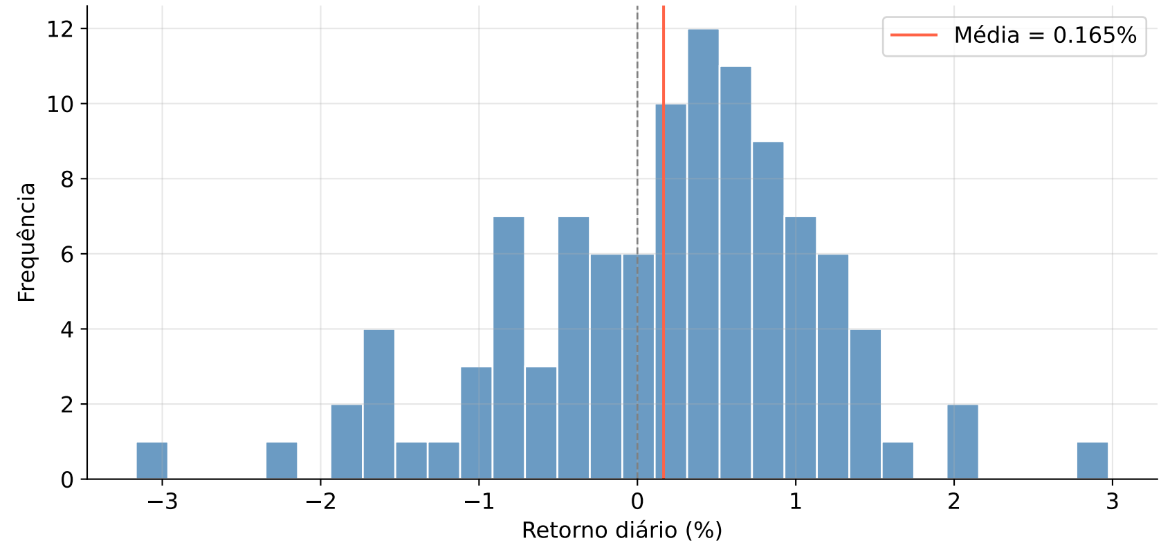
Distribuição dos retornos diários ENERGY
