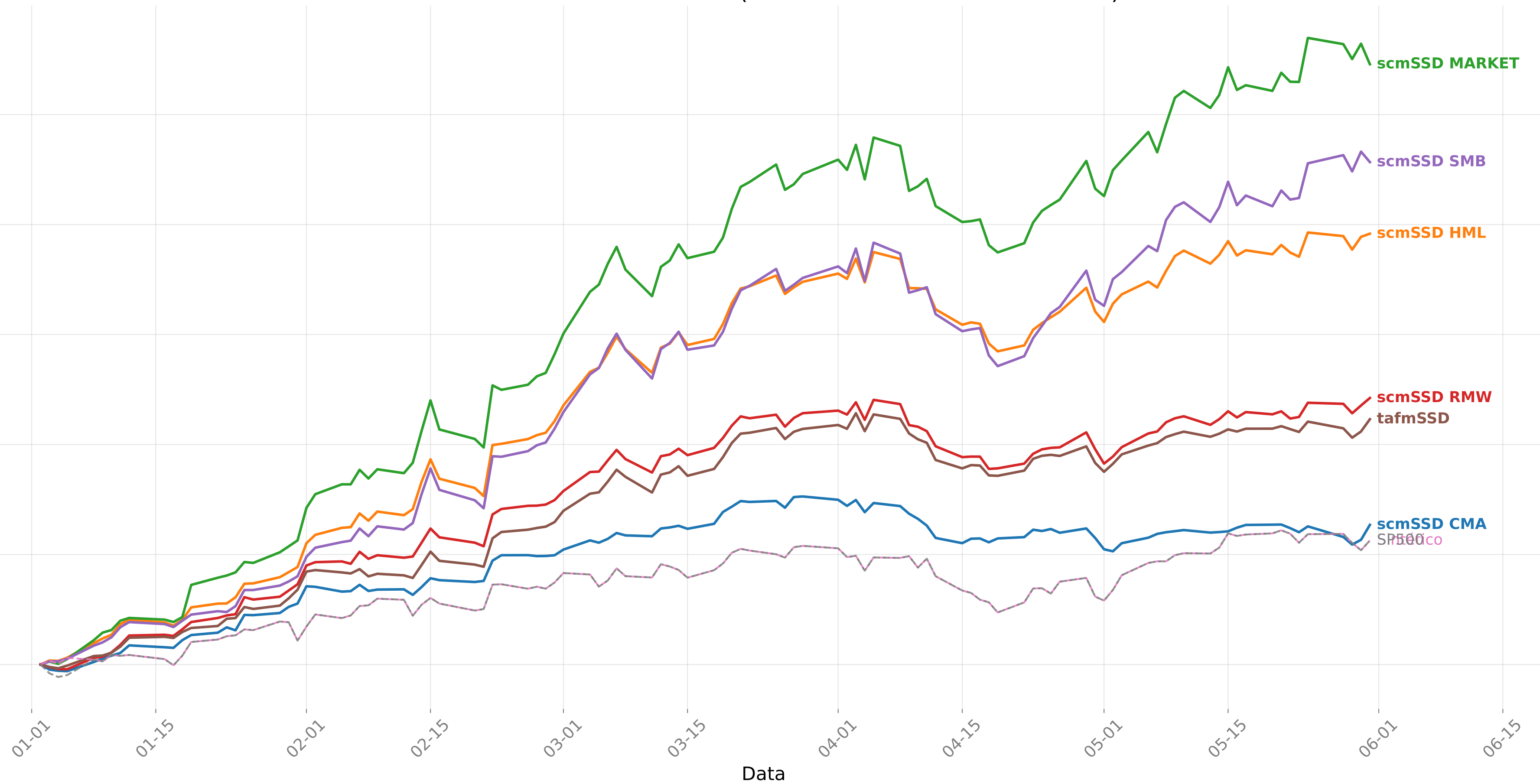
scmSSD fatores vs tafmSSD (benchmarks: sintético + SP500)
