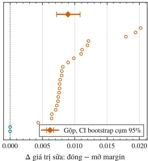
(a) Từng MDP ( n = 25 )
