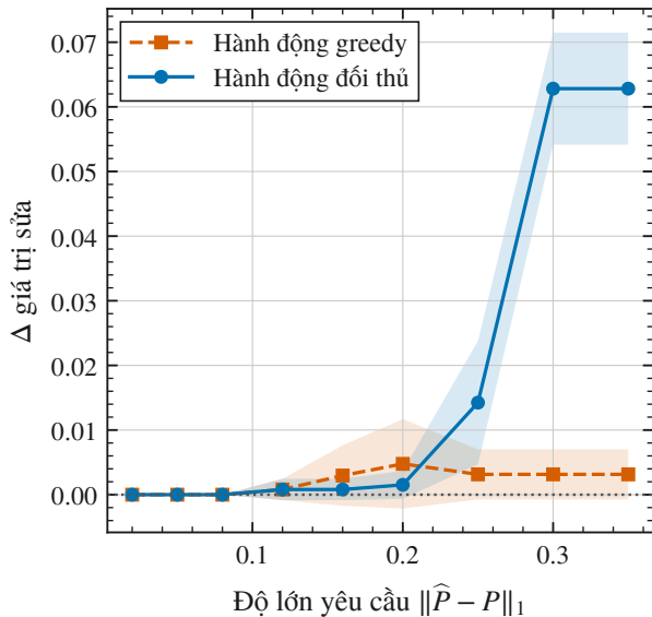
(b) Theo mức sai số
