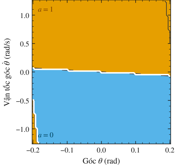
(b) Miền quyết định và đồng mức margin
