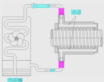
圖 9.2 Cool type I 與冷卻機示意圖
