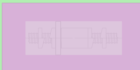
圖4.5 擋塊的安裝實例及不出牙設計
