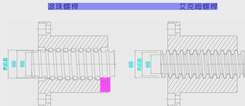
圖2.1 滾珠螺桿與艾克姆螺桿的比較
