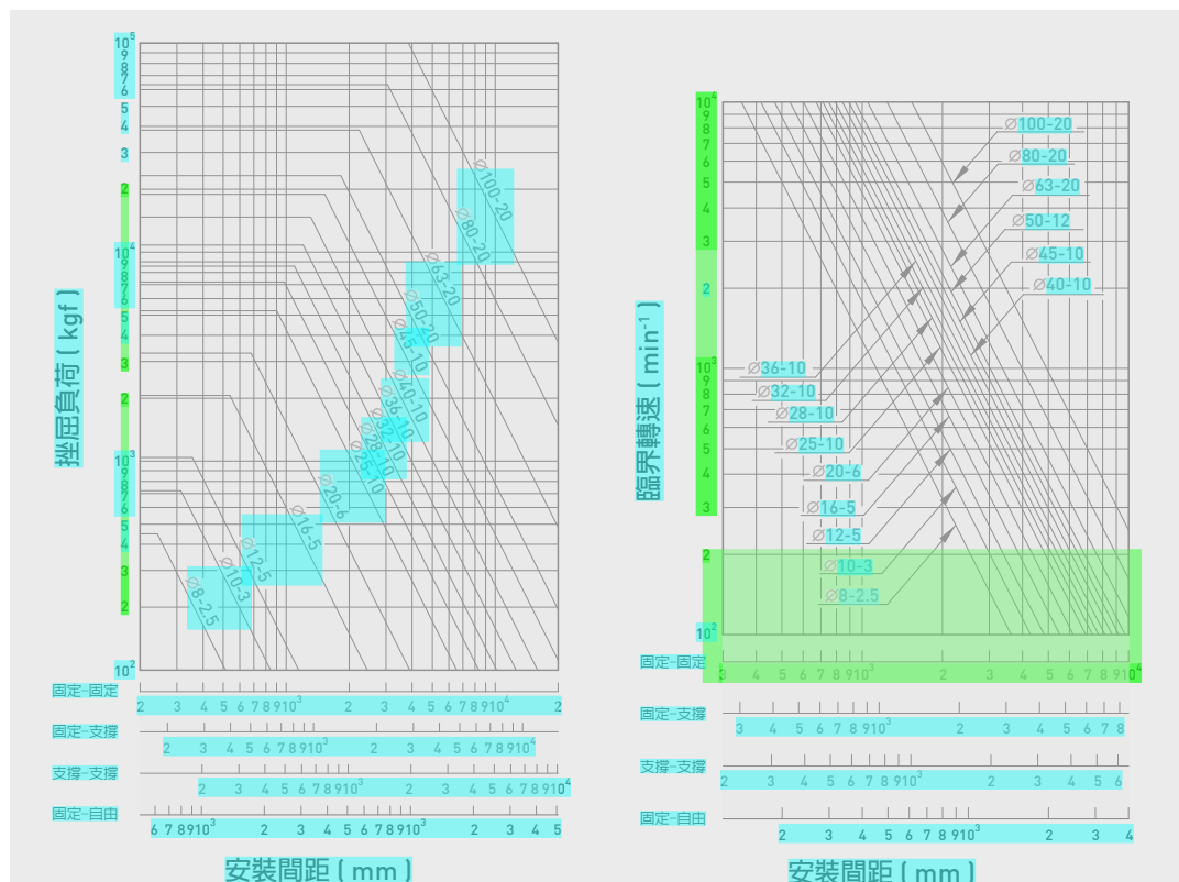
圖4.25 軸徑和安裝間距離相對於挫屈負荷之關係
