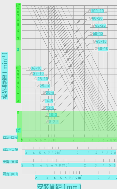
圖4.26 軸徑和安裝間距離相對於臨界轉速之關係
