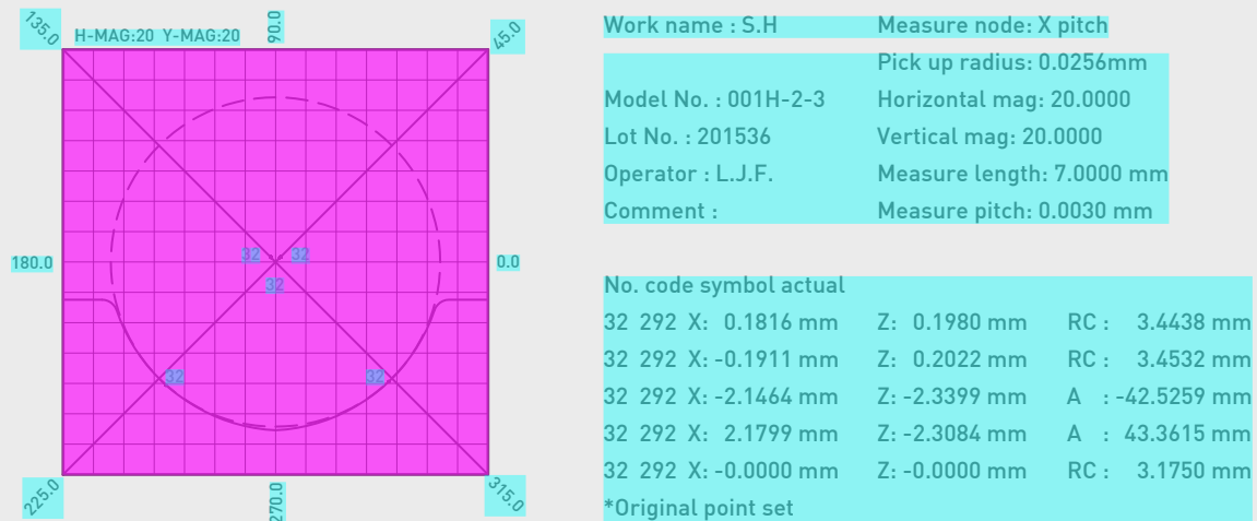
圖2.4 HIWIN滾珠螺桿牙型的檢驗
