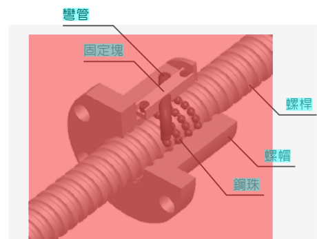
圖3.1 外循環滾珠螺桿
