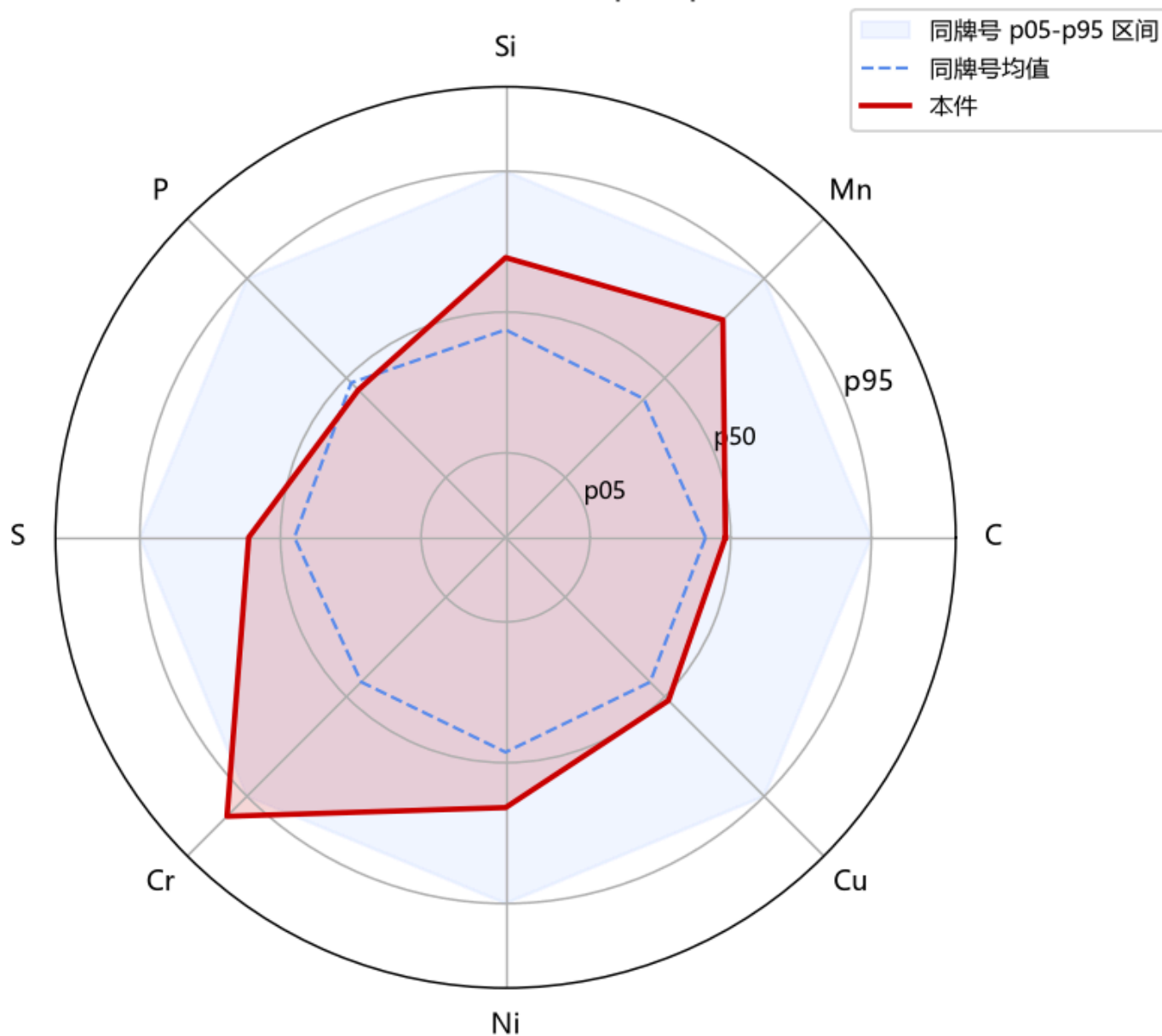
化学成分雷达 (归一化到 p05-p95)
