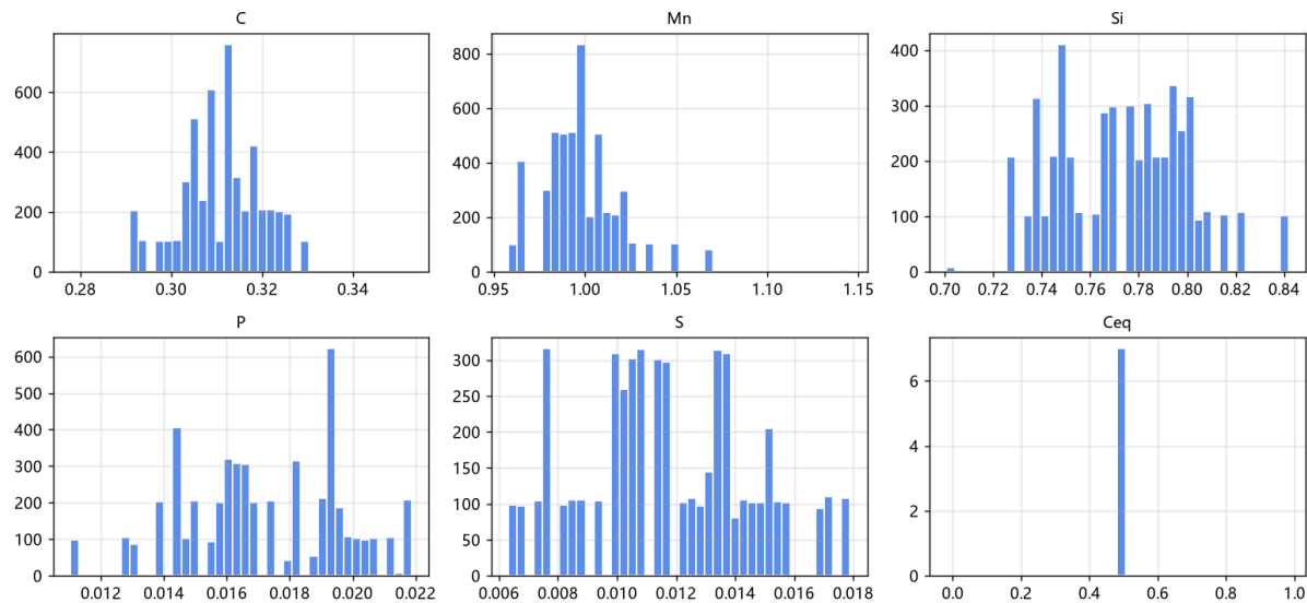
[30MnSi] 化学成分分布
