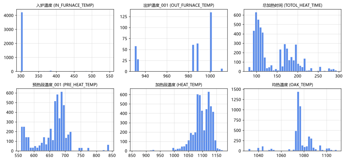
[ML08AI] 加热工艺分布
