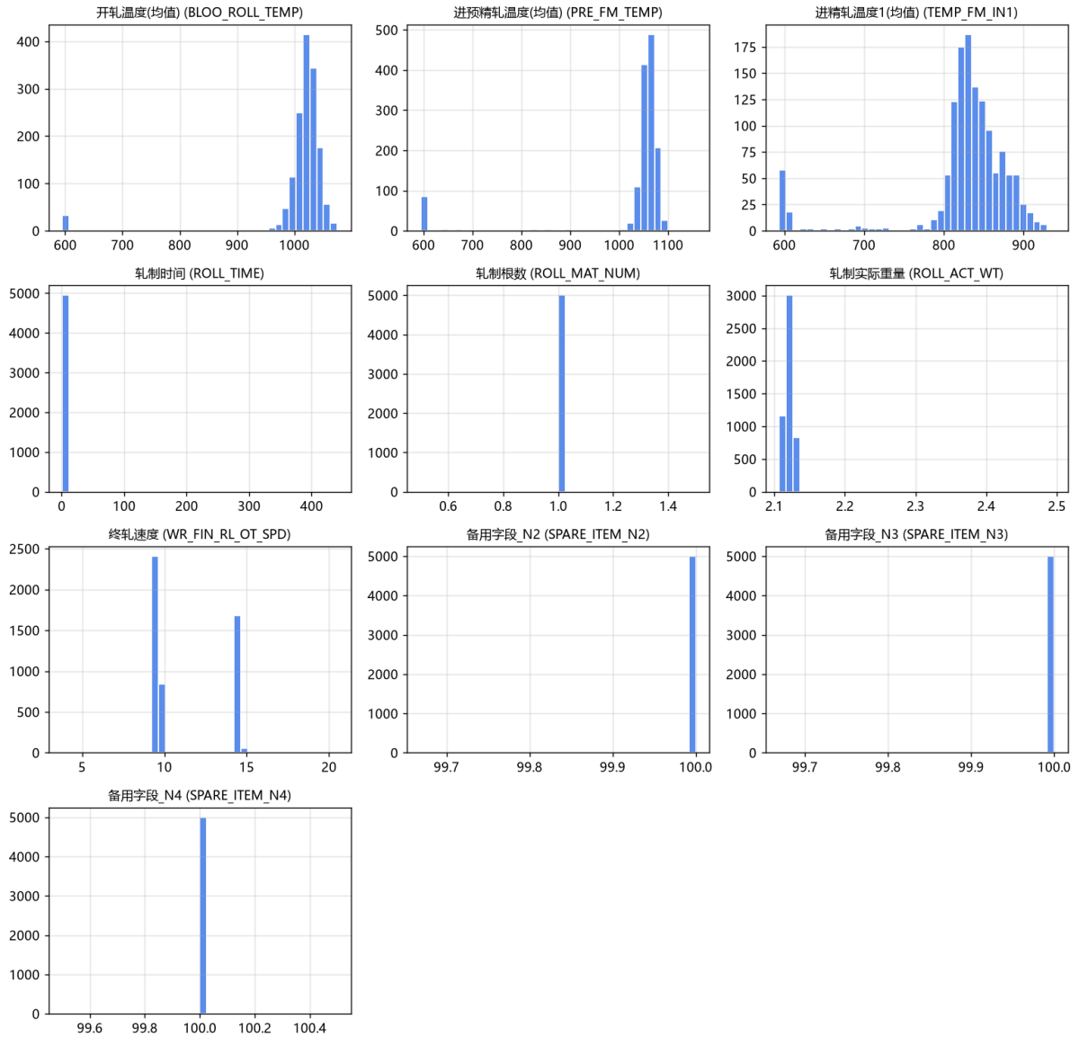
[HRB400E] 轧制工艺分布
