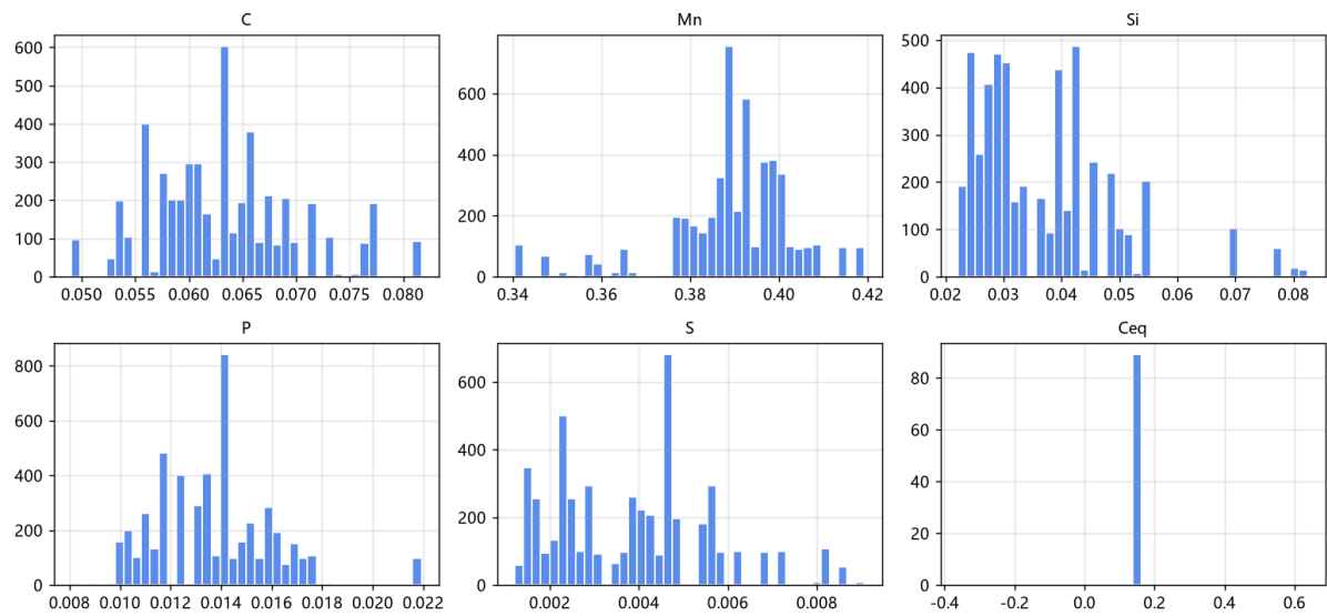
[ML08AI] 化学成分分布
