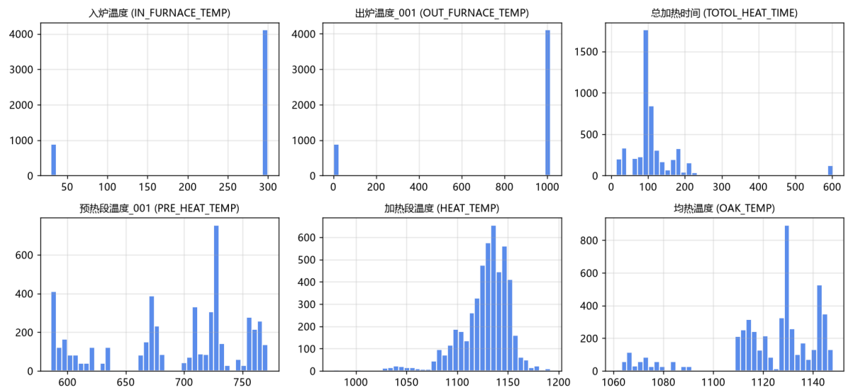
[30MnSi] 加热工艺分布
