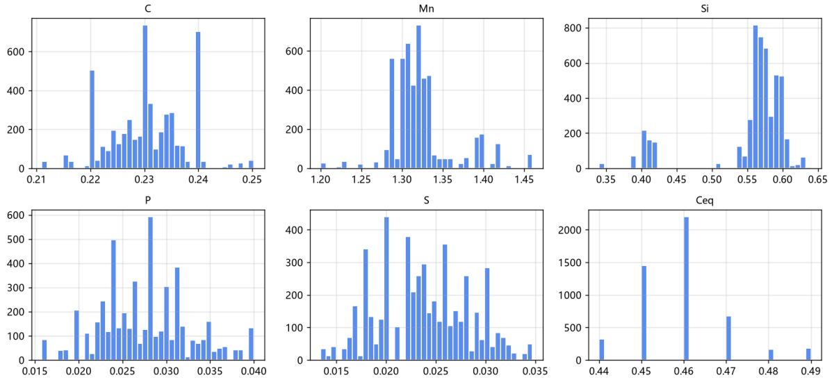
[HRB400E] 化学成分分布
