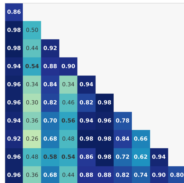
LIBERO-10
