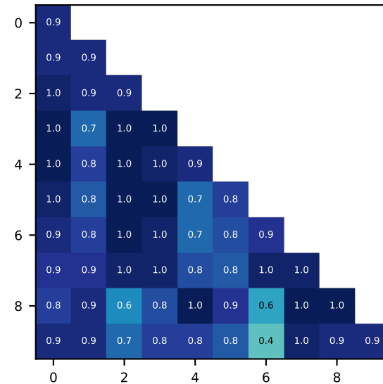
BC-Diffusion
