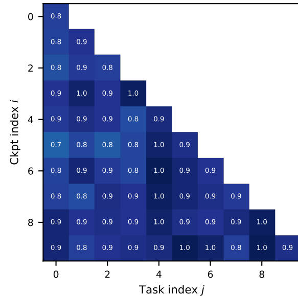
Pi0
