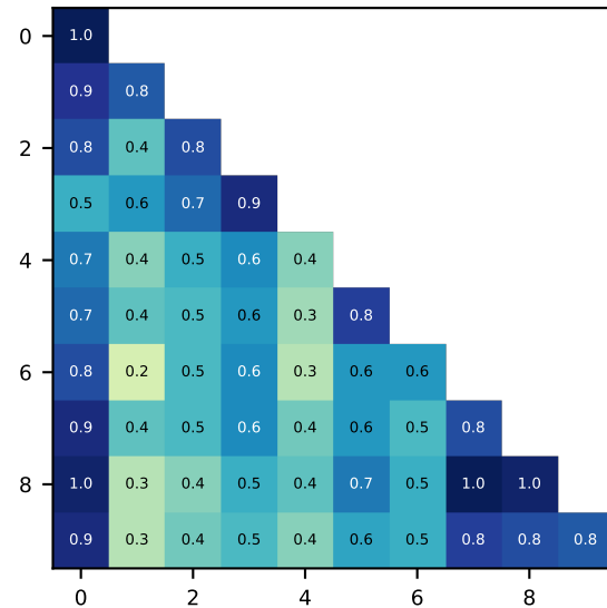
BC-ViT
