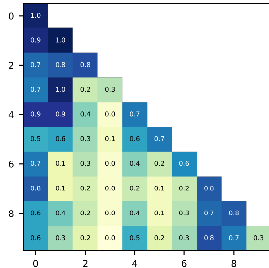
BC-ViT
