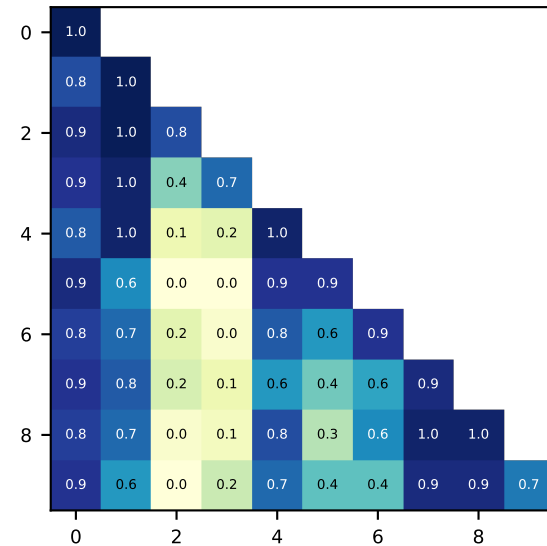
BC-Diffusion
