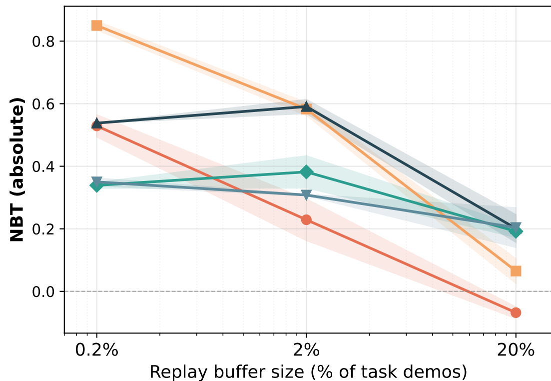
LIBERO-10: Absolute NBT
