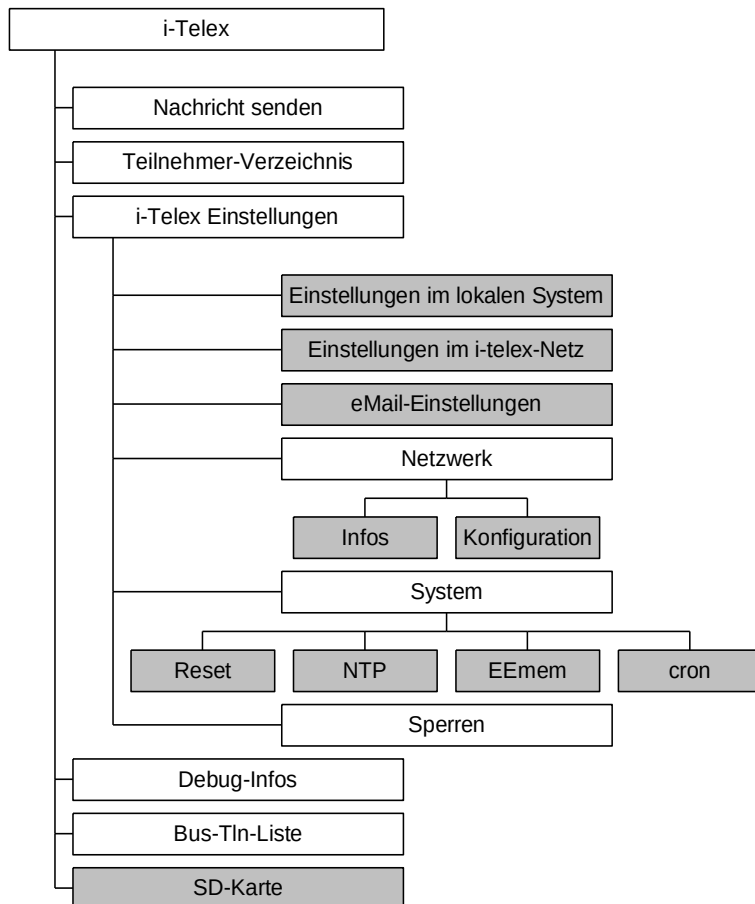
Abbildung 4: Menübaum
