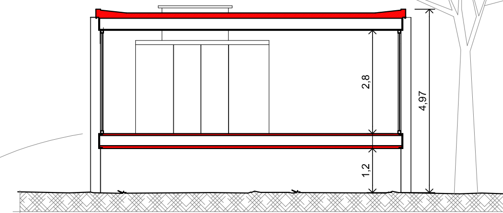
CORTE A-B ESC:1-100
