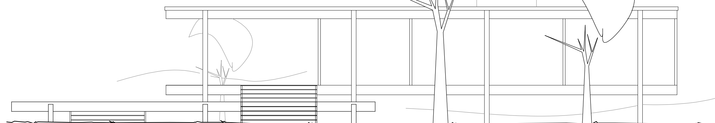
VISTA SUR ESC:1-100
