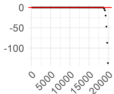
(e) p=100, n=100
