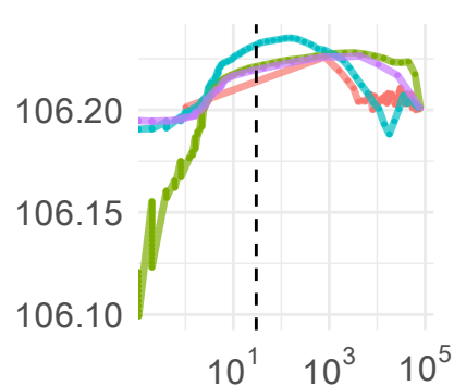
(l) p=400, n=800
