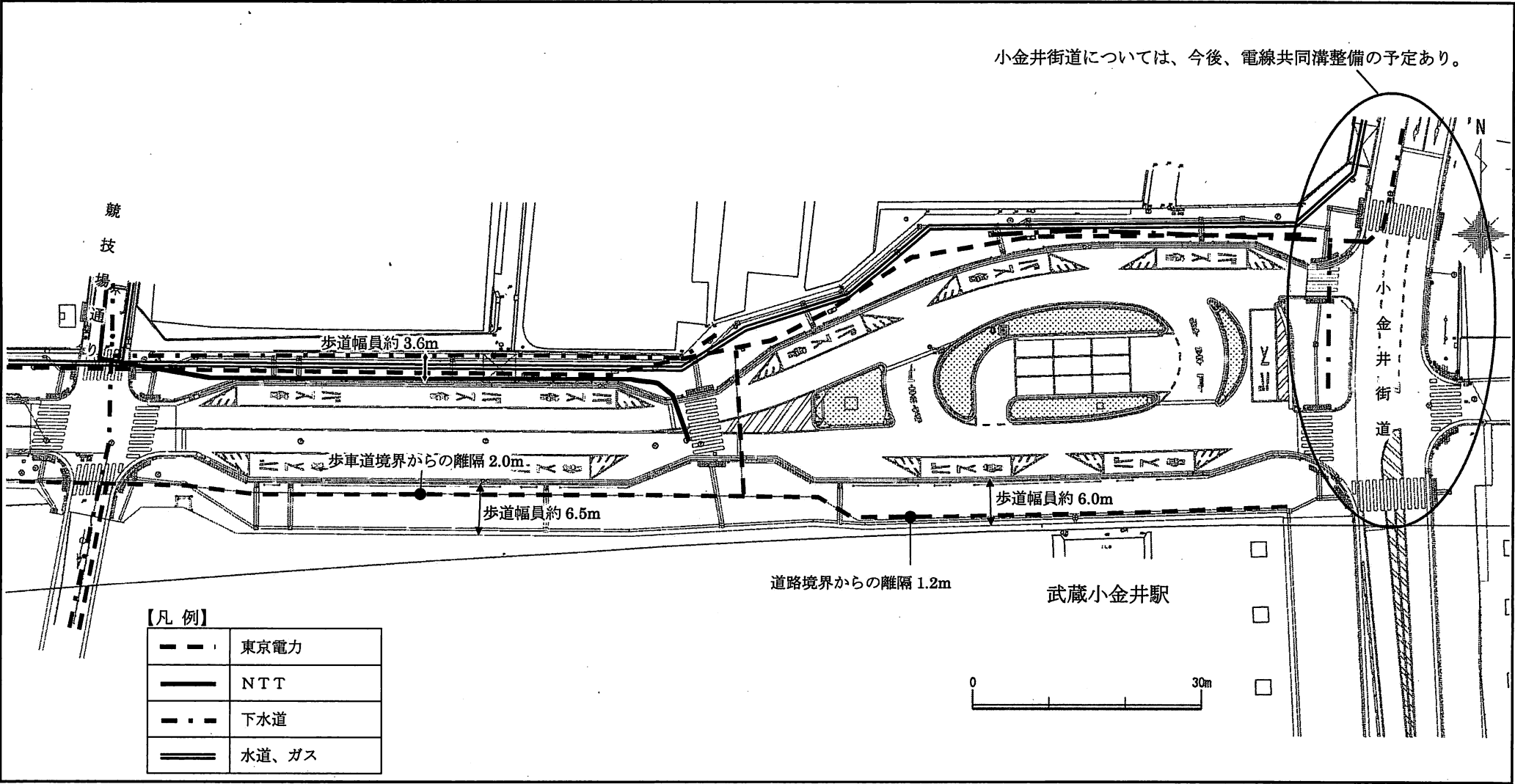
武蔵小金井駅北口における地下埋設物位置図
