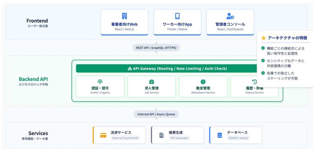
図 2.2: システムアーキテクチャ概要（主要サービス間の疎結合構成）
