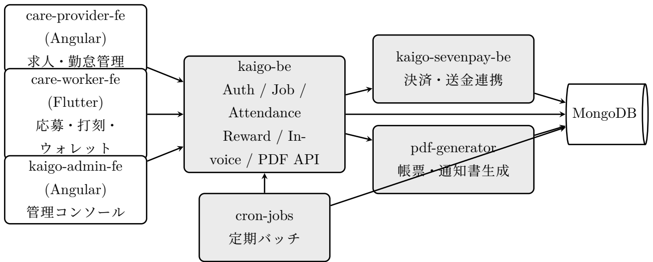
図 1.7: システムアーキテクチャ概要（主要サービス間の疎結合構成）
