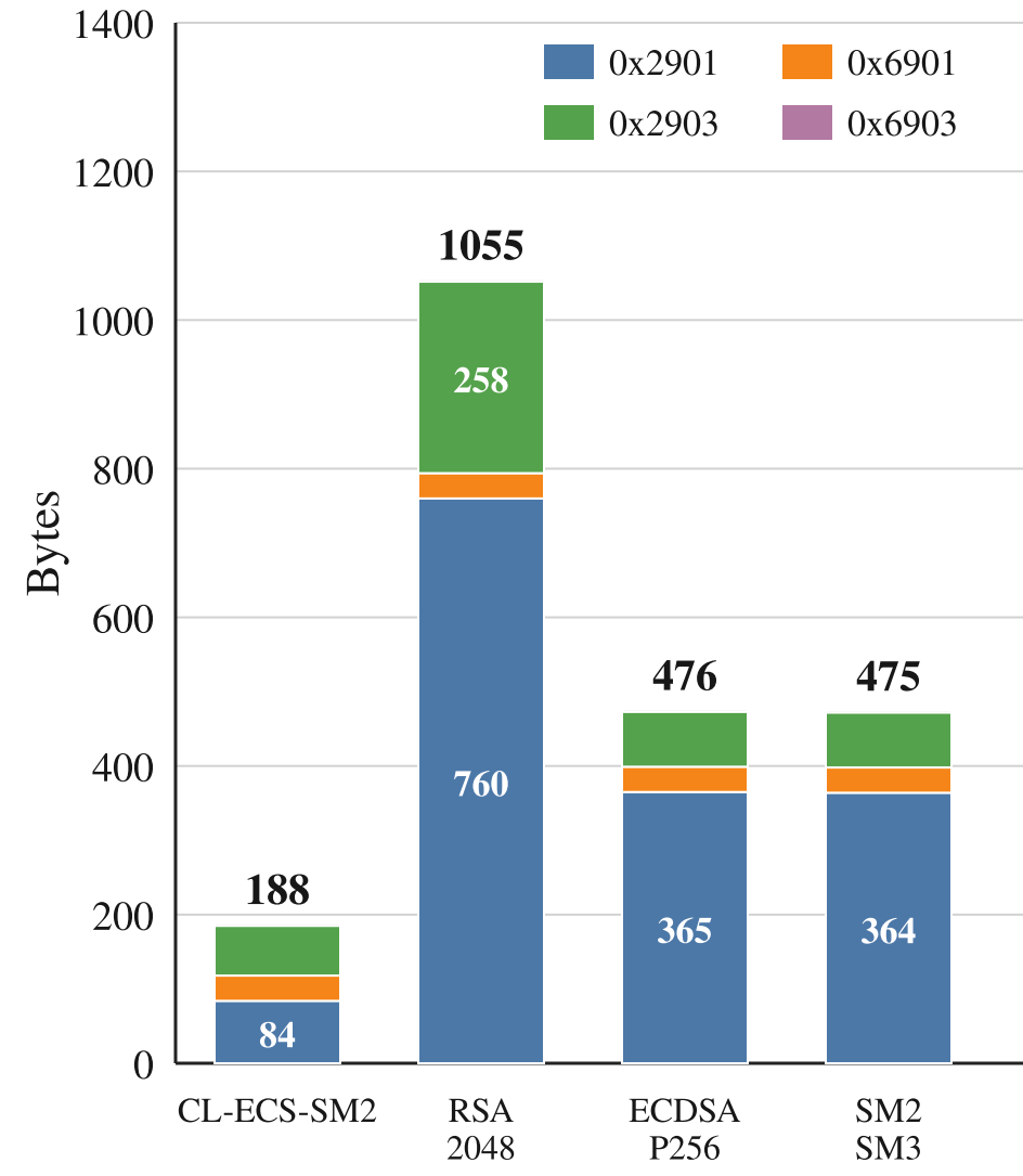
(b) UDS payload size
