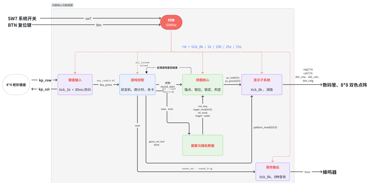
图 2-1 系统总体框图（第一层：7 个功能子系统，含模块功能与模块间信号传递关系）
