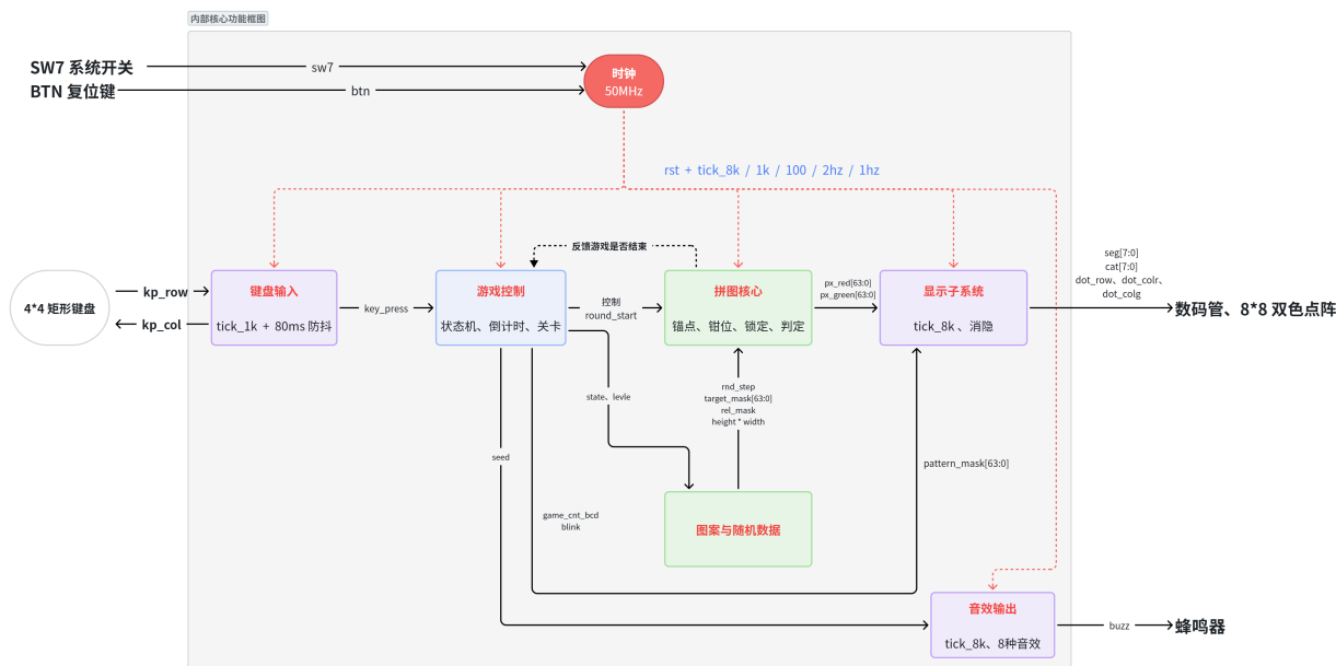
图 2-1 系统总体框图（第一层：7 个功能子系统，含模块功能与主要信号）
