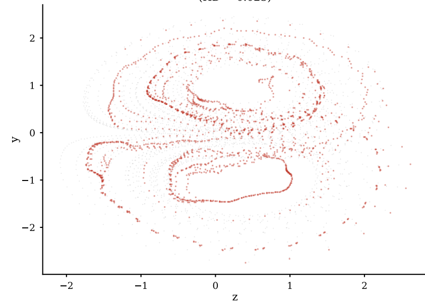
Lorenz (HD = 0.023)
