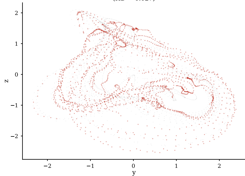
Halvorsen (HD = 0.027)
