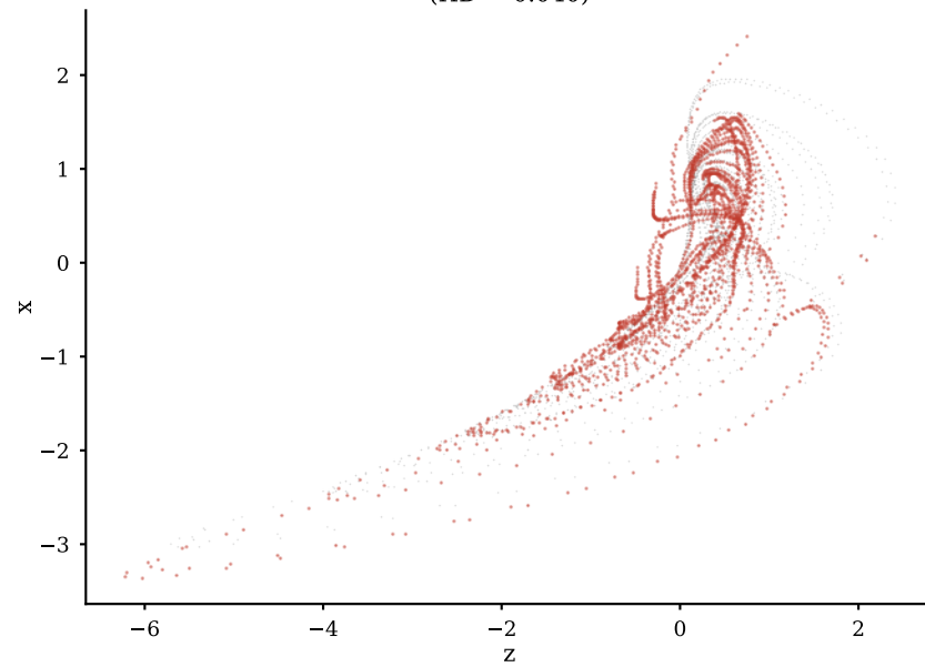
SprottR (HD = 0.040)
