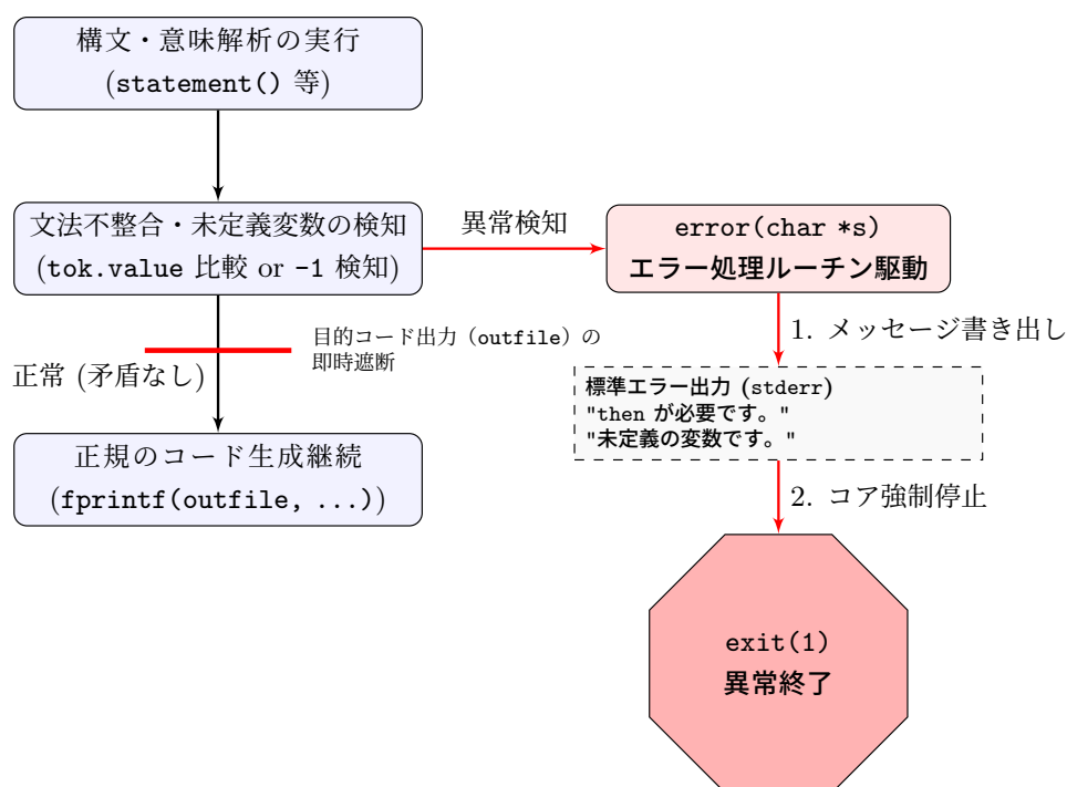
図 9 エラー検知時におけるコンパイル処理の遮断と終了
