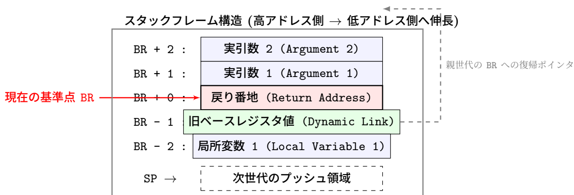
図 8 再帰呼び出し時におけるスタックフレームの構造図
