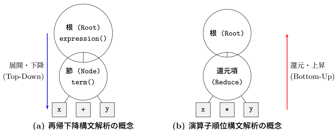
図7 構文解析手法の違いによる走査方向と構文木構築の概念図
