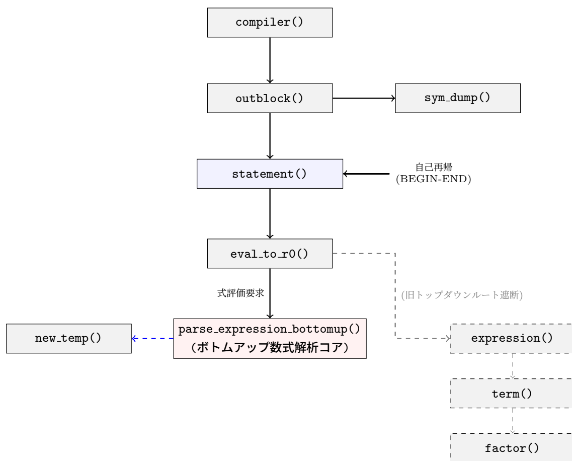
図 11 コンパイラ内部の関数コールツリーとボトムアップ差し替えにともなう依存関係図
