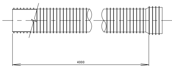
側 面 図
