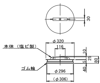
内蓋
