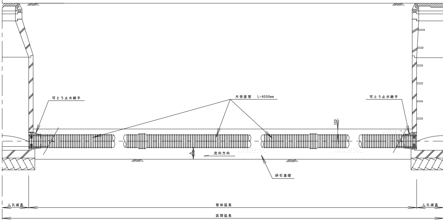
A—A 断 面 図
