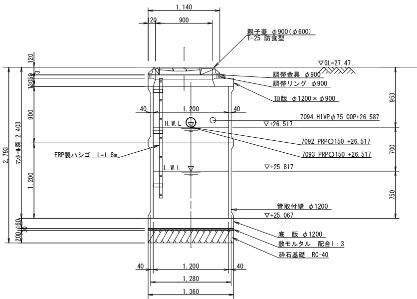
B-B断面図
