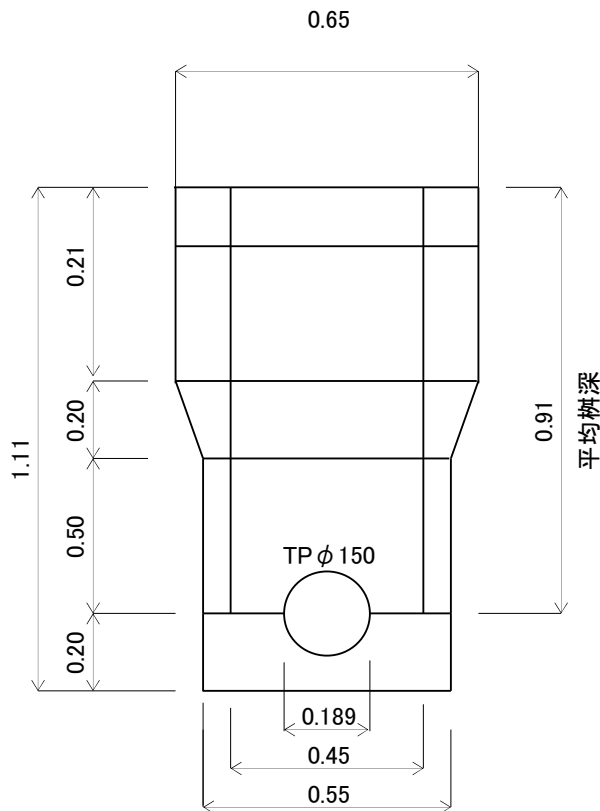
断面図
