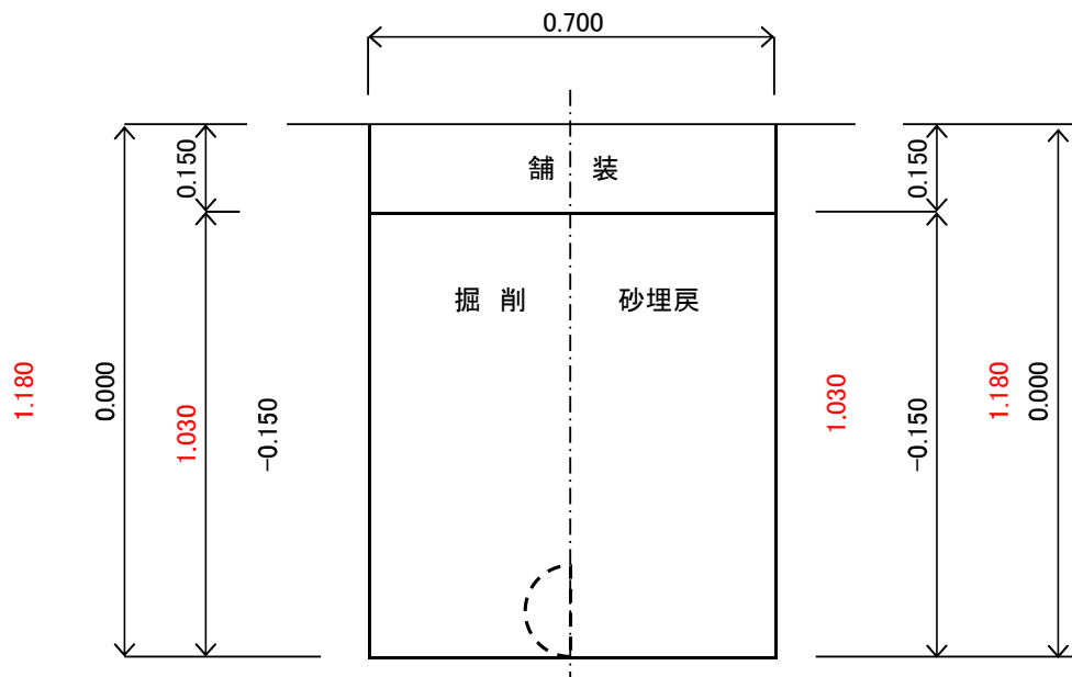
←掘削 | 埋戻→
