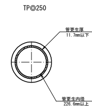
管更生詳細図 S=1:10
