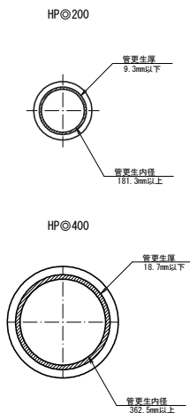
管更生詳細図 S=1:10
