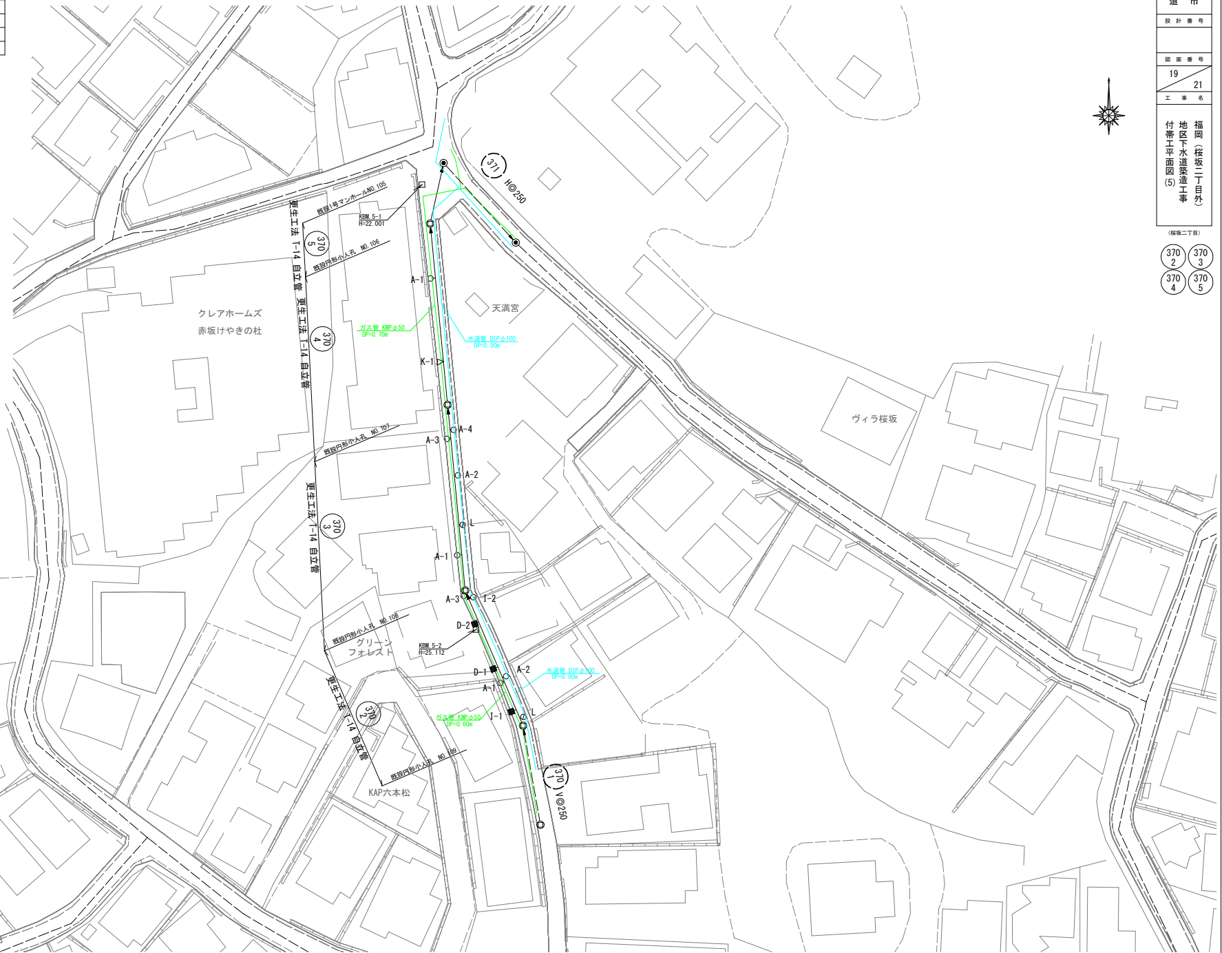
付帯工平面図 (5) A1図面 S=1:300 A3図面 S=1:600
