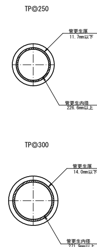
管更生詳細図 S=1:10
