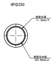
管更生詳細図 S=1:10
