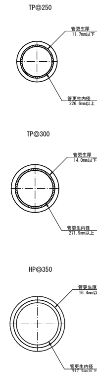
管更生詳細図 S=1:10
