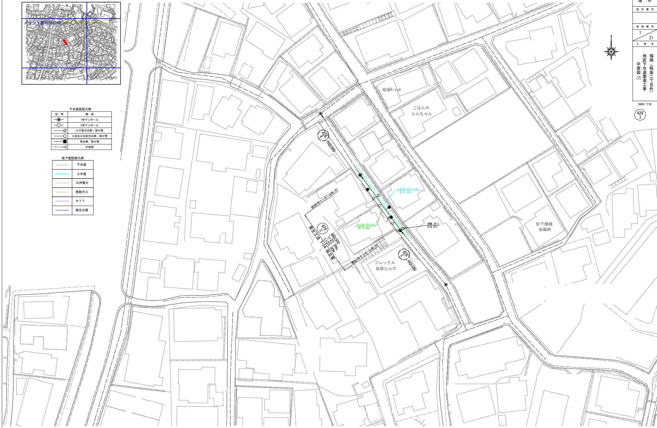
平面図(7)
