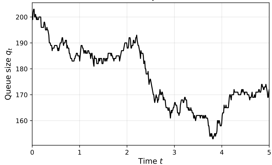
Queue Dynamics
