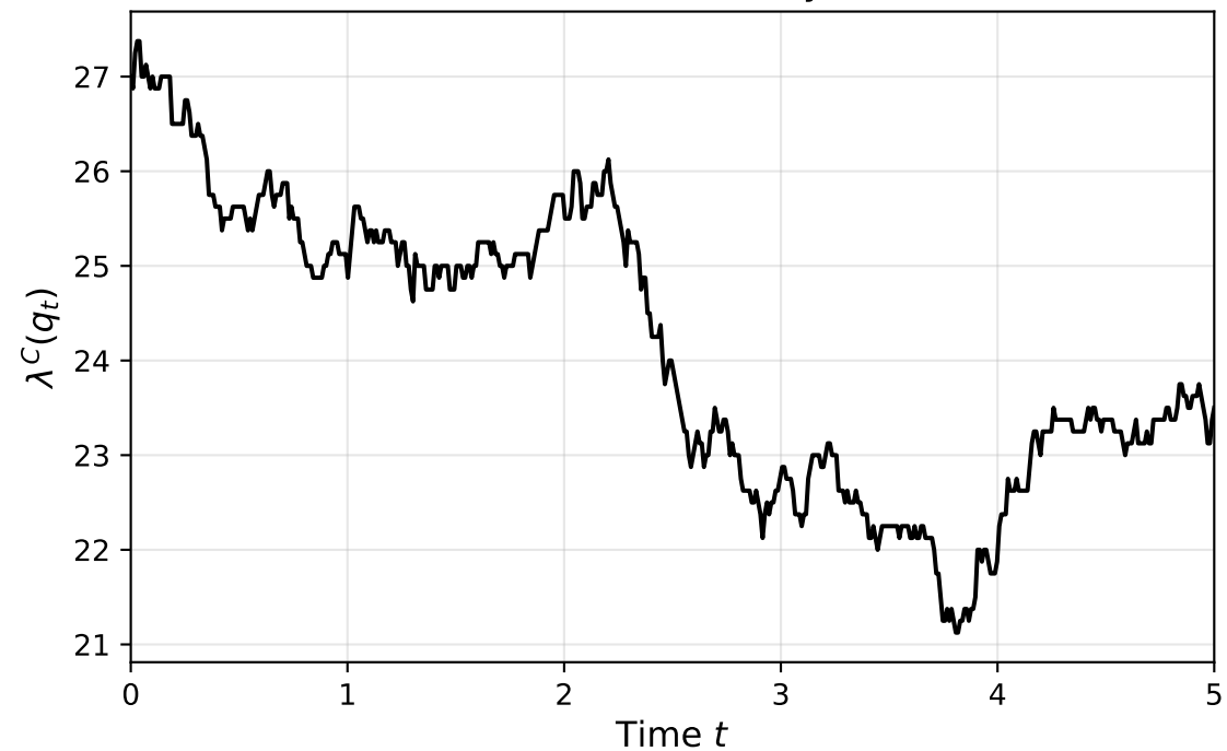
Queue Dynamics
