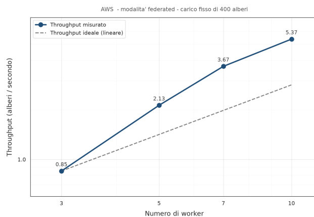
Throughput addestramento del sistema distribuito
