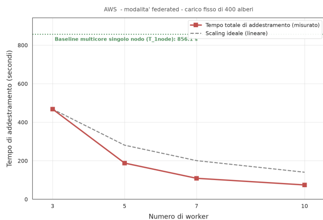
Strong scaling: tempo di addestramento a carico costante
