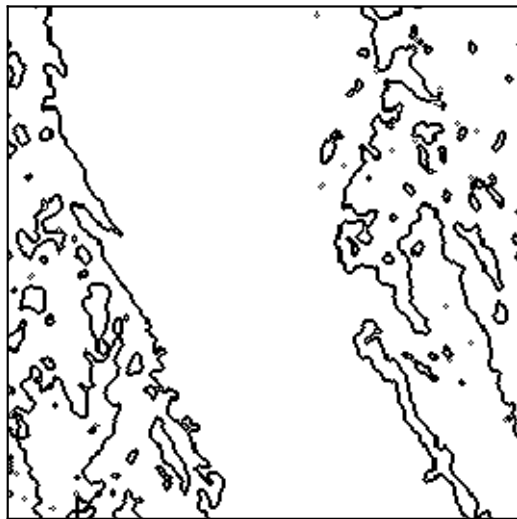
[6 7 0 2 1 4 3 5]: D=1.53
