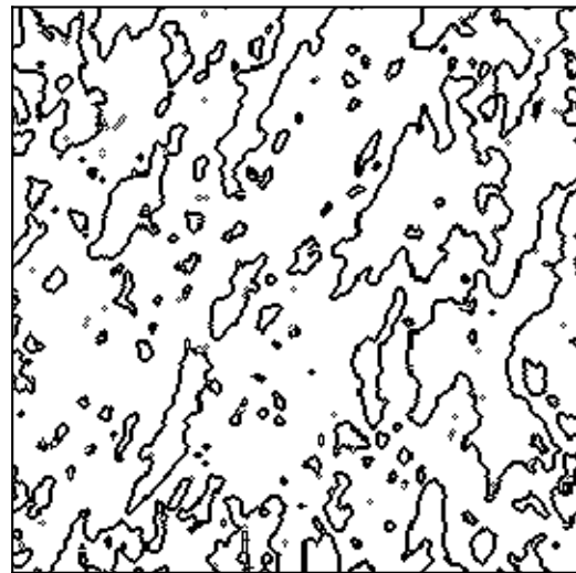
offset +1: D=1.64
