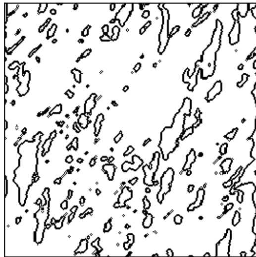
\sigma=16250374 : D=1.58
