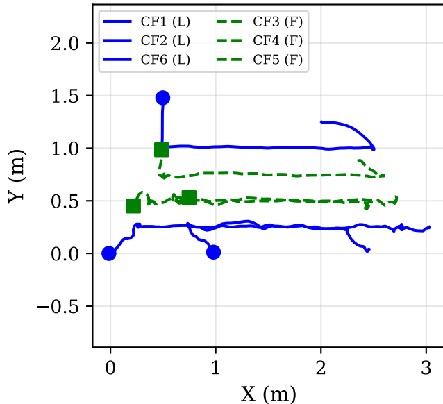
(b) Actual Trajectories (Vicon)
