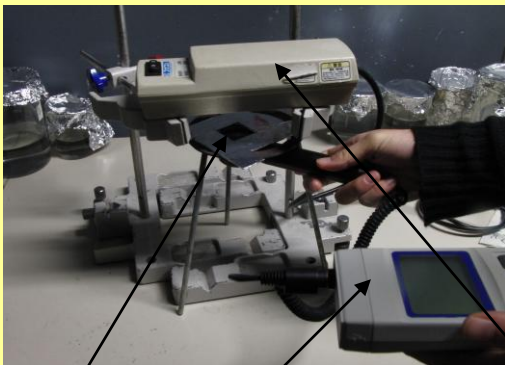
試料 UV メーター UV ライト
