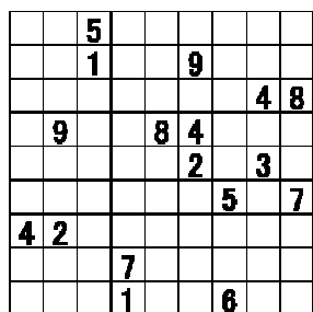
図1 通常ナンプレ ヒント数17
