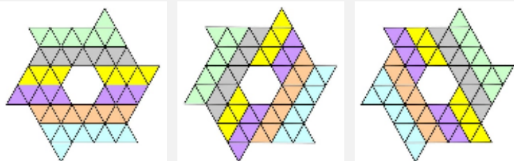
図3 星形ナンプレ 列
