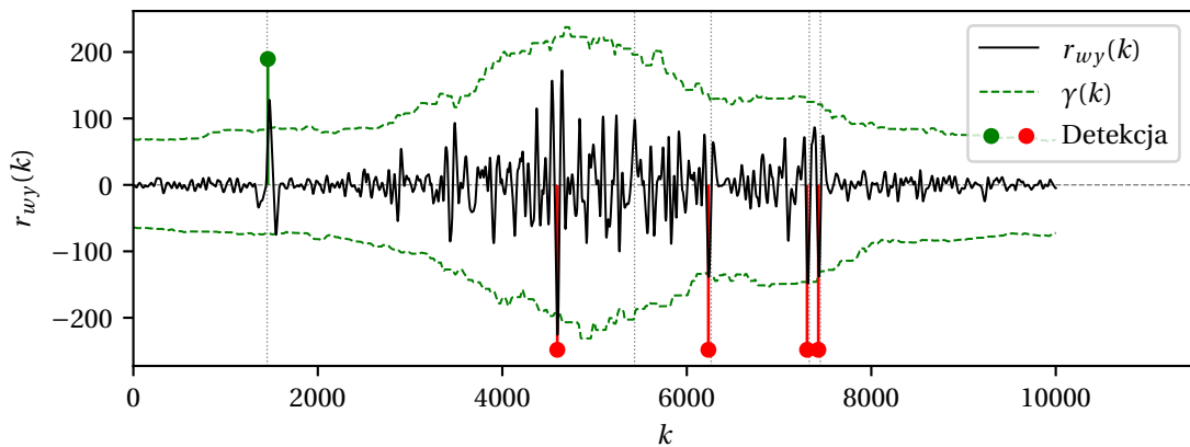
(c) Algorytm z progowaniem adaptacyjnym
