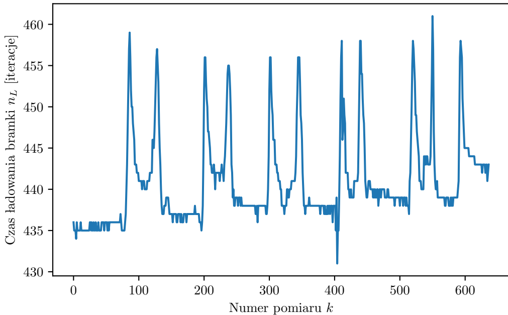
Przebieg wyjścia czujnika
