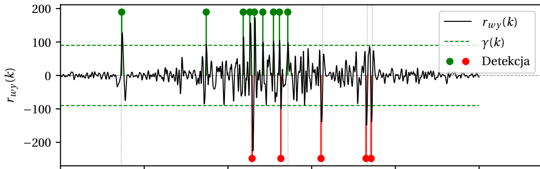
(c) Algorytm z progowaniem adaptacyjnym
