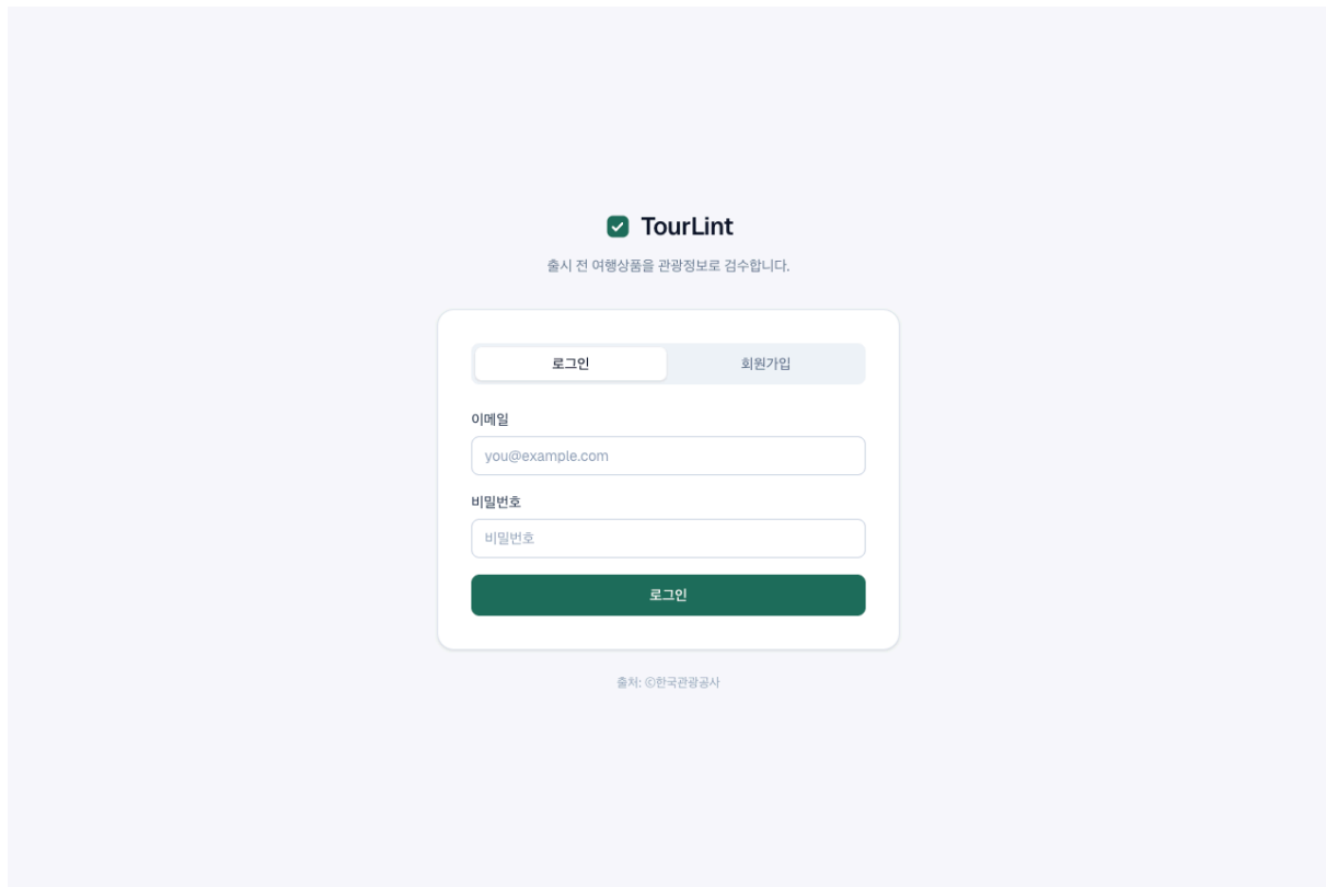
로그인 화면
