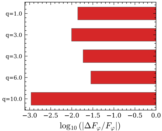
(b) F_\varphi relative error
