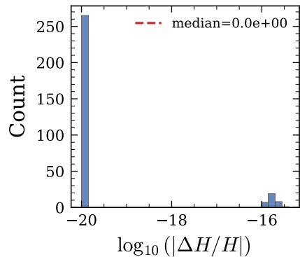
(d) \partial_r H (FD vs analytical)
