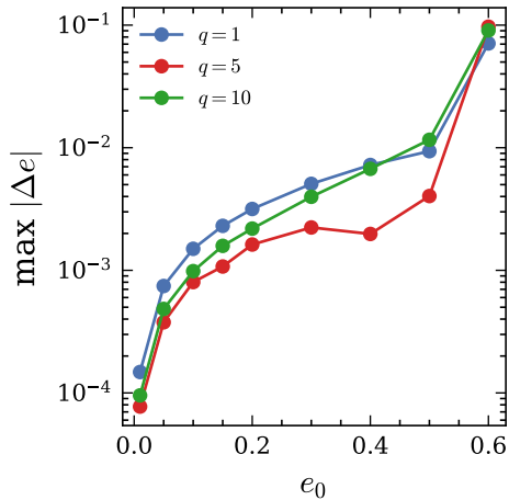
(b) Eccentricity error
