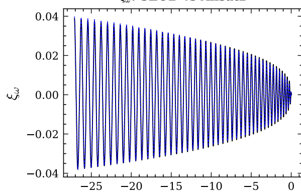
\xi_\omega : SEOB vs Ansatz
