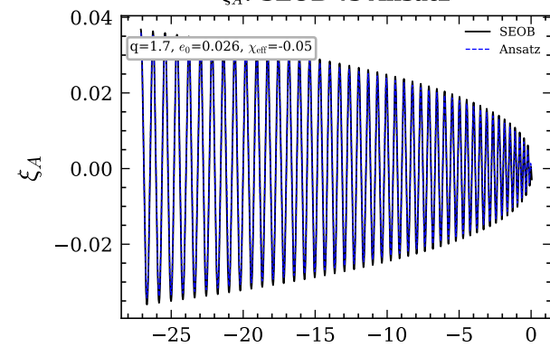
\xi_A : SEOB vs Ansatz
