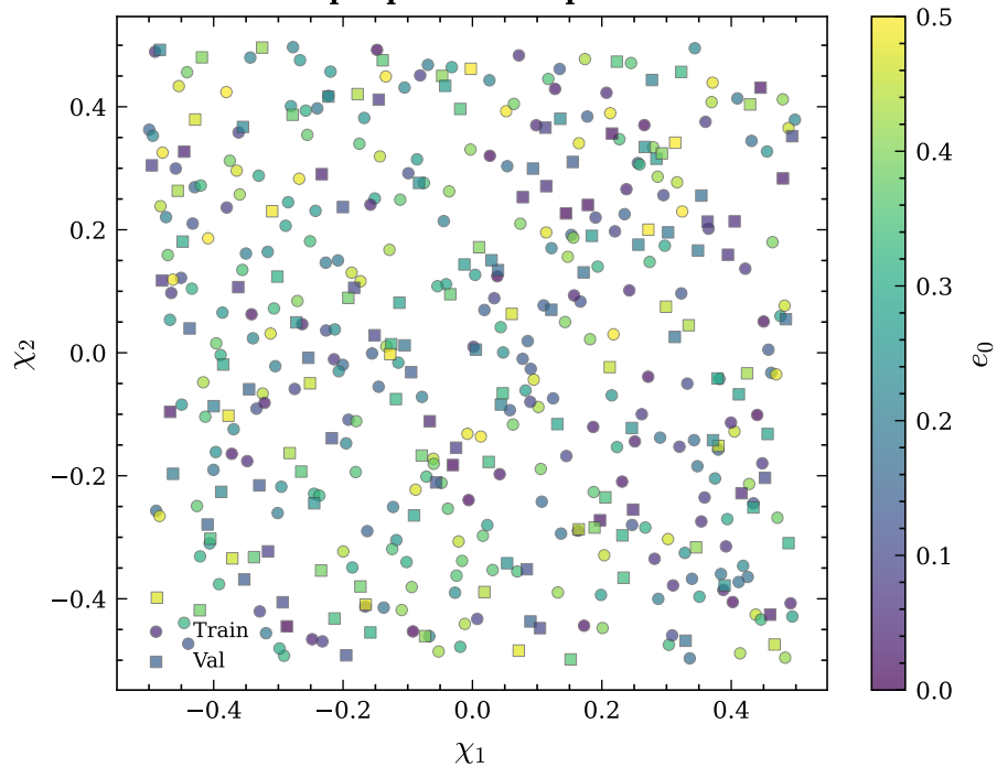
Spin parameter space
