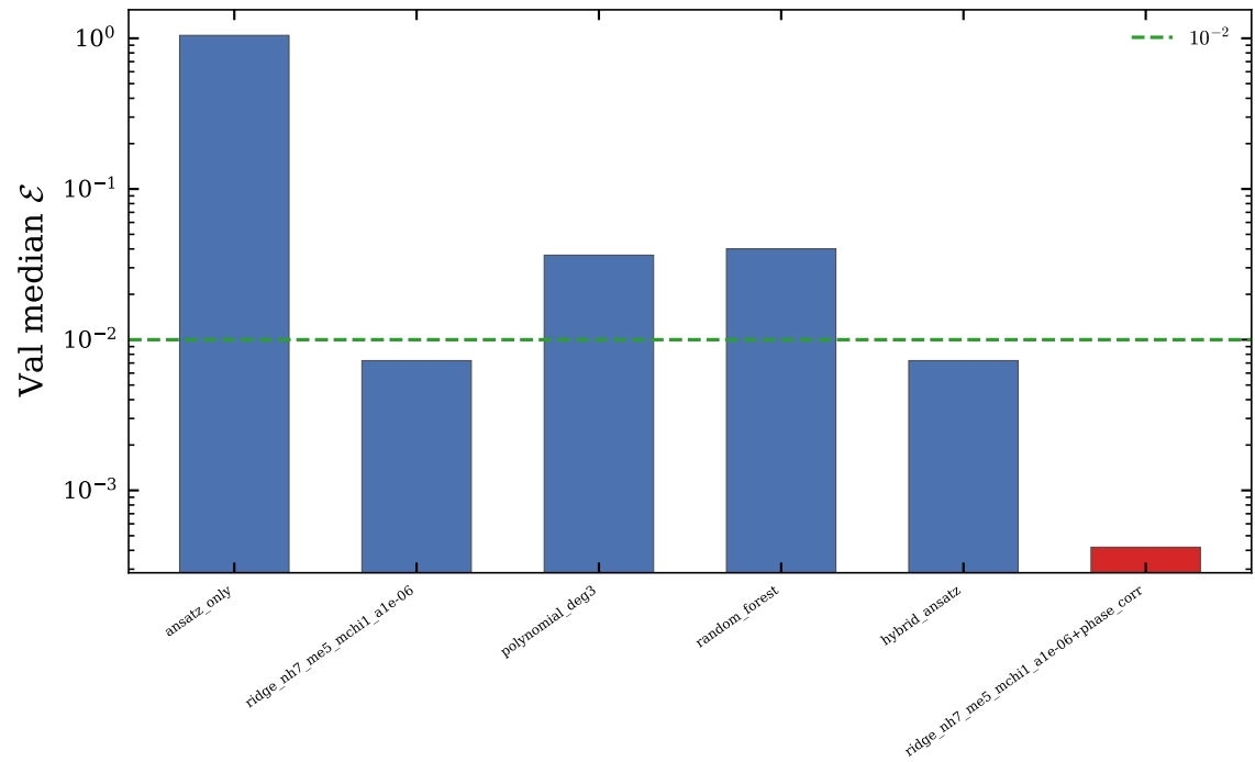
\mathcal{E} progress
