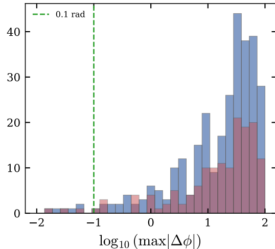
ansatz_only: dephasing
