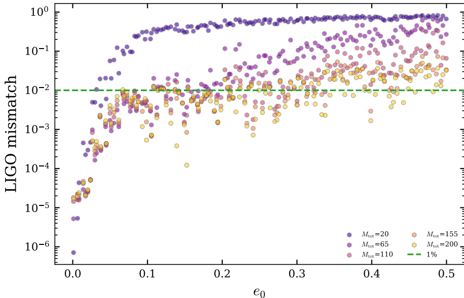
ansatz_only: LIGO MM vs e_0
