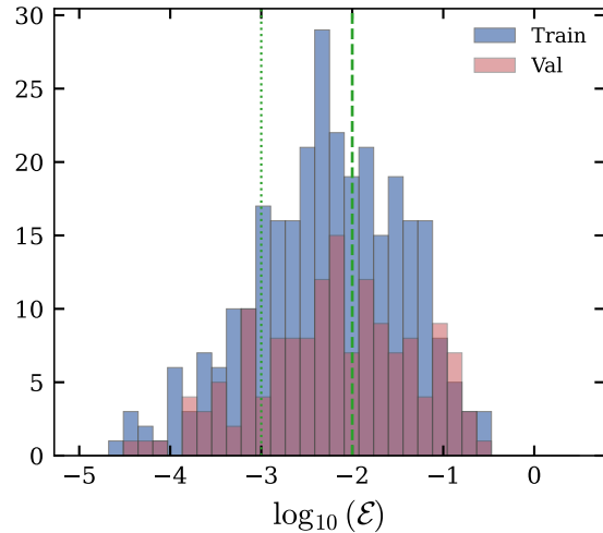
hybrid_ansatz: \mathcal{E}
