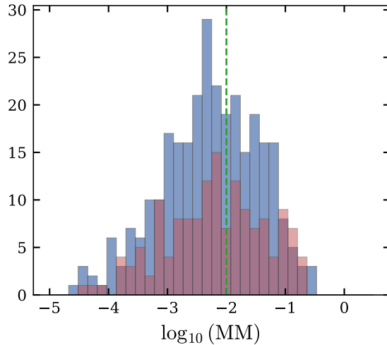
hybrid_ansatz: MM
