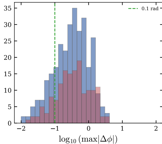
hybrid_ansatz: dephasing
