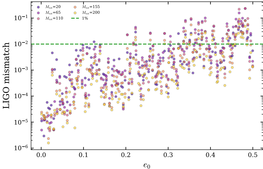
hybrid_ansatz: LIGO MM vs e_0
