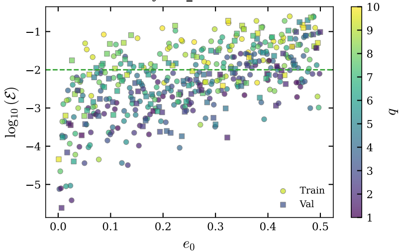
hybrid_ansatz
