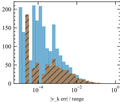
xgboost pn
