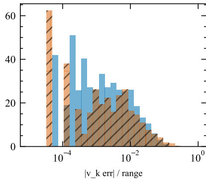
xgboost pn
