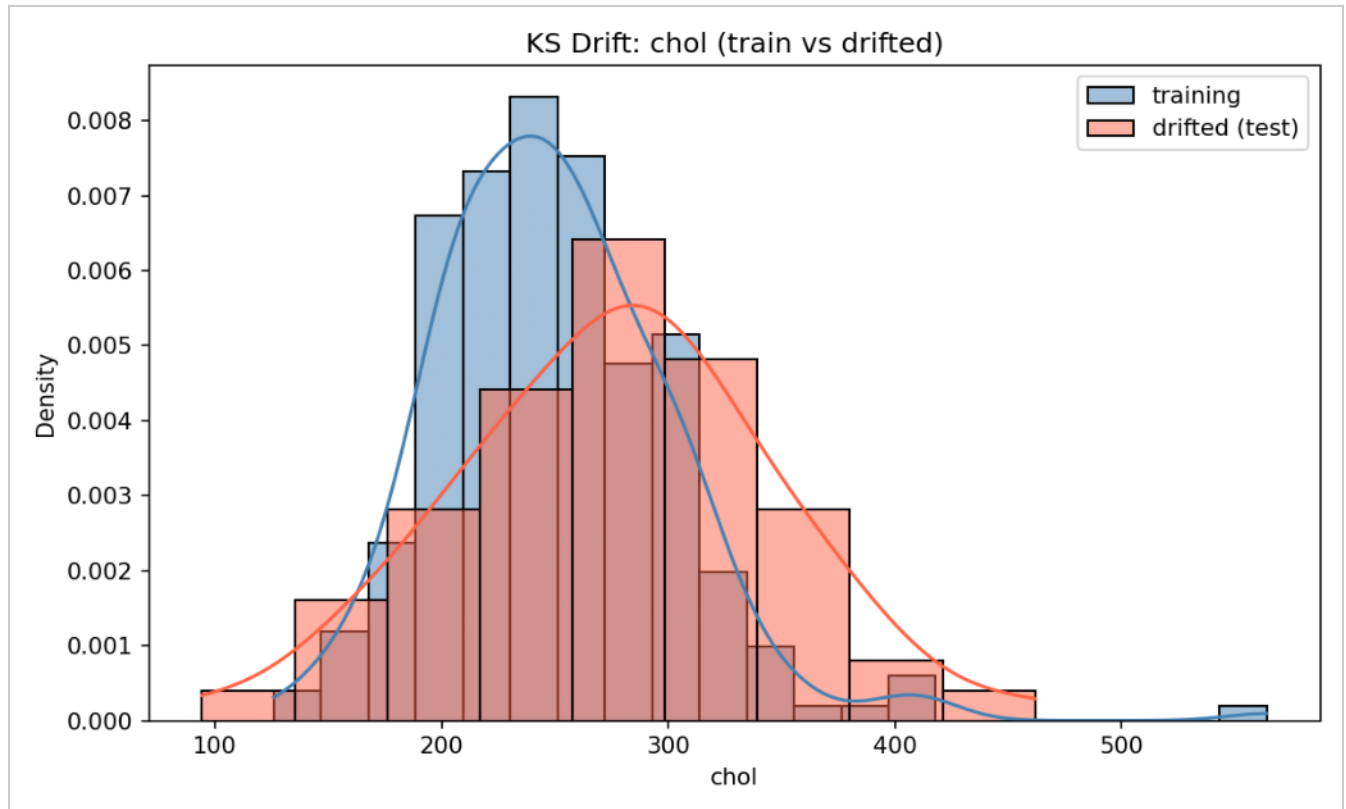
그림 5. KS 드리프트 (chol)
