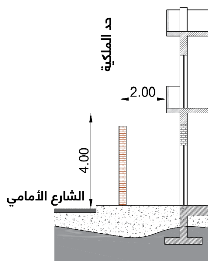
شكل رقم (٤١) البروزات
