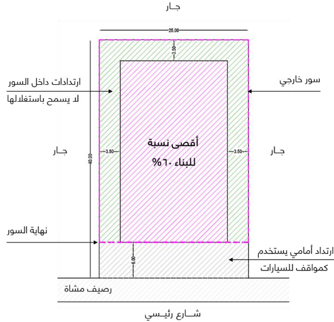
شكل رقم (١٠٢) الارتدادات بالورش المهنية ضمن المناطق الصناعية (ص١)
