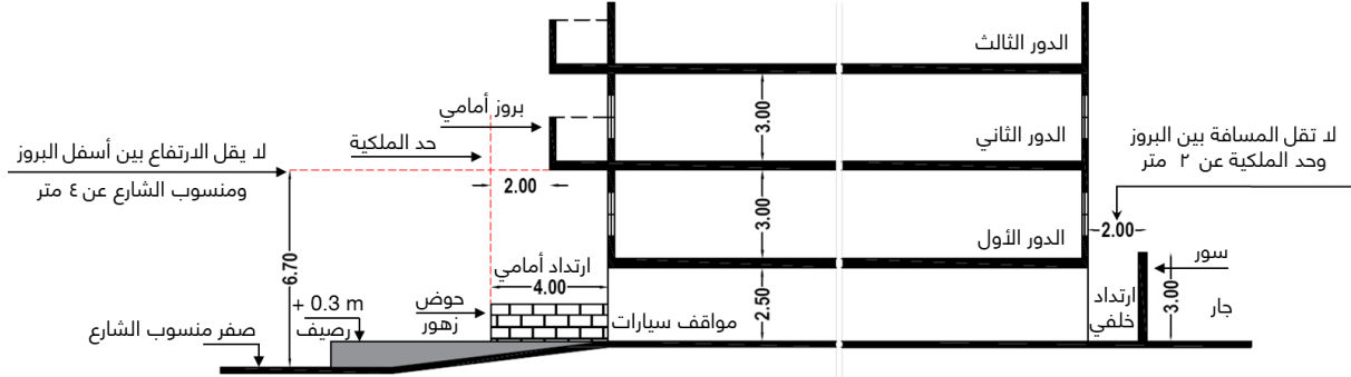
شكل رقم (٩٠) ارتفاع البروز وارتداده عن حد الملكية
