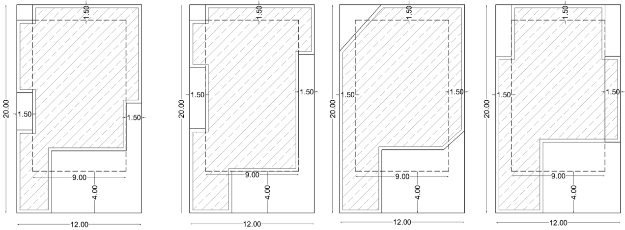
شكل رقم (٦٤) نسبة البناء للدور الأرضي بما فيها الملاحق الأرضية بمناطق الفيلات
