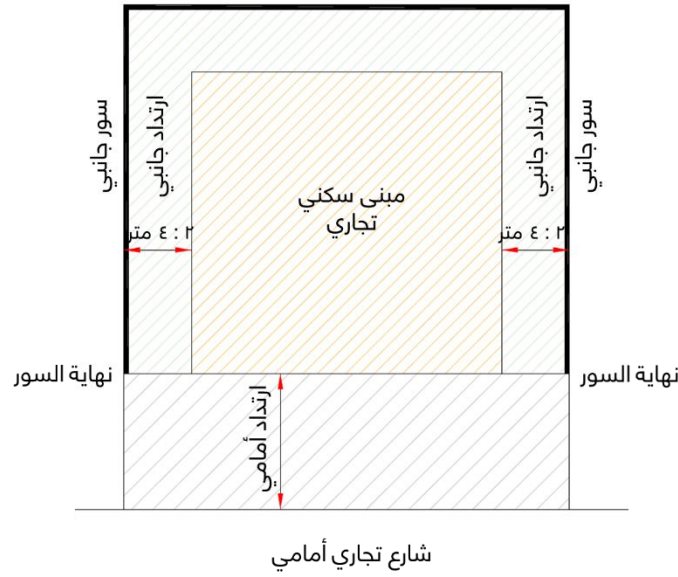
شكل رقم (٣٦) يوضح نهاية الأسوار الجانبية مع الدترداد الأمامي
