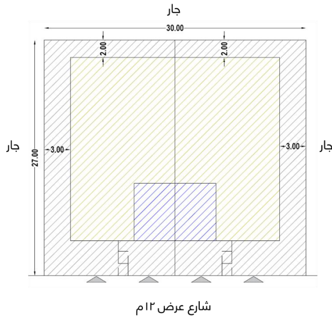
شكل رقم (٦٠) نموذج يوضح مداخل لأربع وحدات سكنية (دور أرضي ودور علوي)
