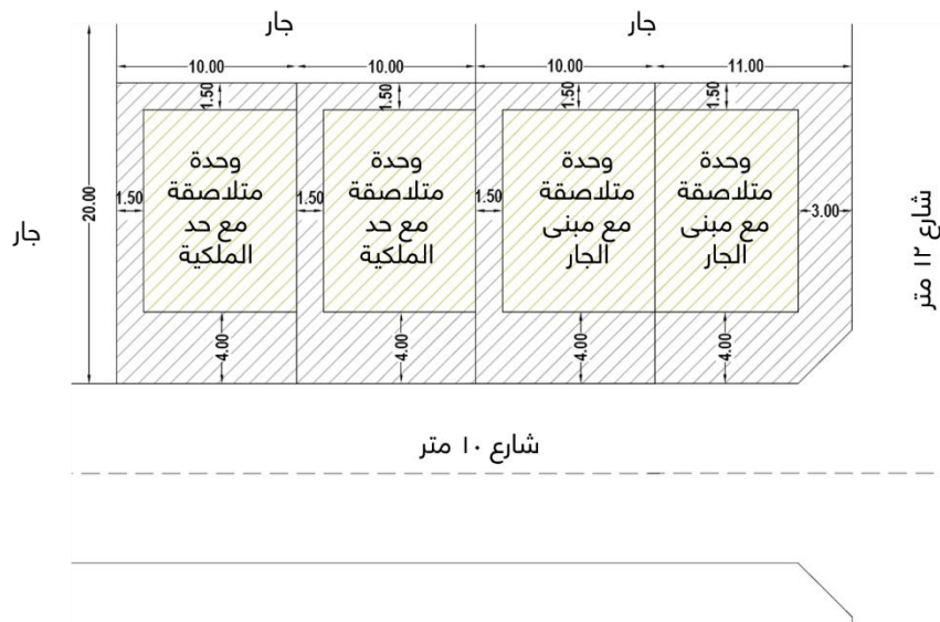
شكل رقم (06) الدمج بين الوحدات المتلاصقة من جهة واحدة مع مبنى أو مع حد الملكية
