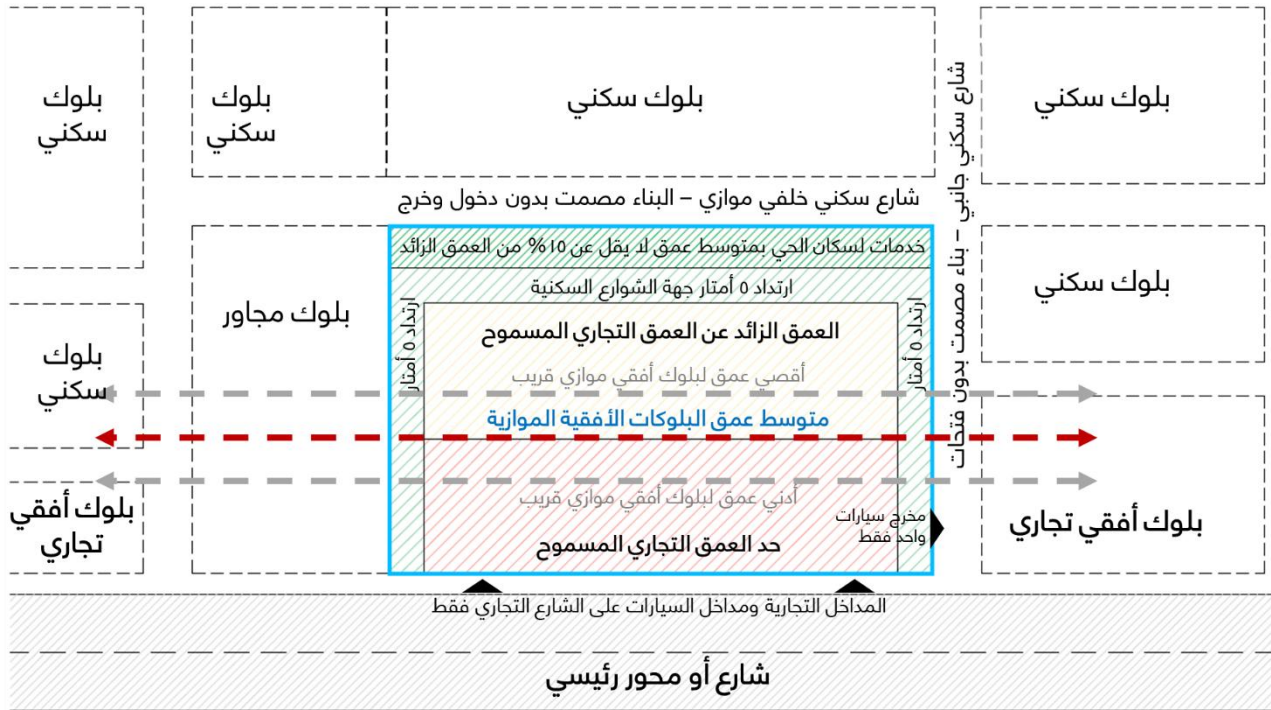
شكل رقم (٤٨) شكل توضيحي لموقع محاط بشوارع وجوار
