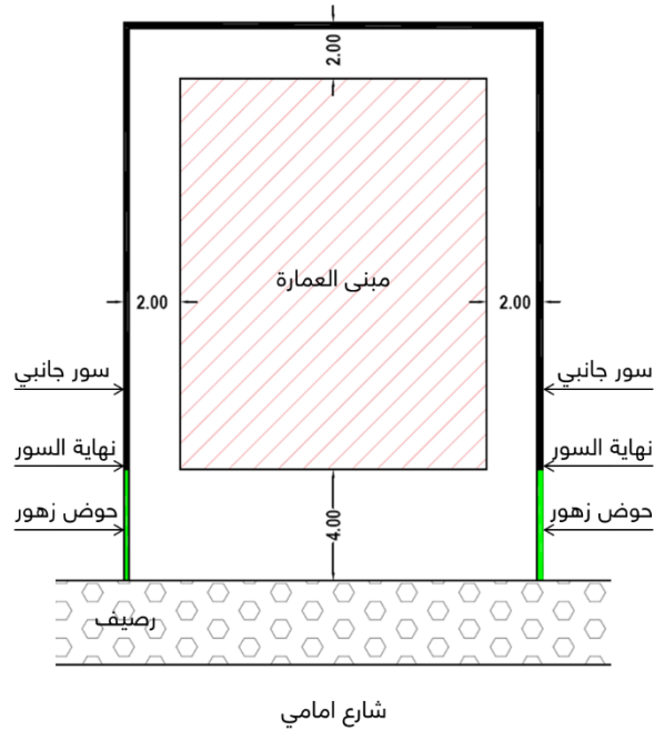
شكل رقم (٧٩) نهاية الأسوار الجانبية مع الارتفاع الأمامي
