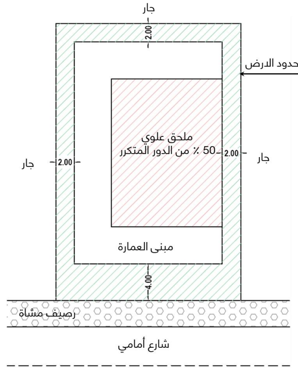
شكل رقم (٨) موقع الملحق بالنسبة للمبنى
