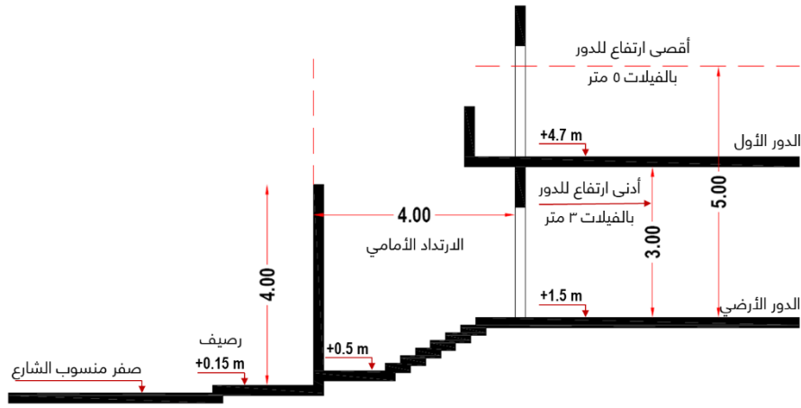
شكل رقم (٦٦) قطاع يوضح ارتداد وارتفاع مباني الفيلات
