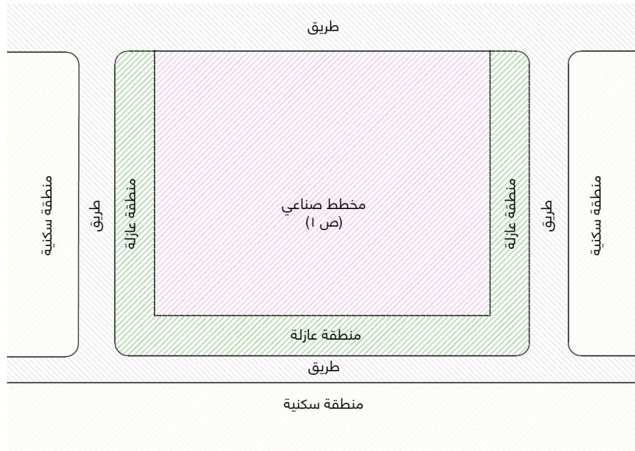
شكل رقم (٩٥) طريقة عزل المناطق الصناعية (ص ١) عن الاستعمالات السكنية المجاورة لها
