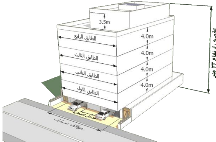
شكل رقم (٧٤) يوضح أقصى عدد للدوار والارتفاعات بمناطق العمارات السكنية
