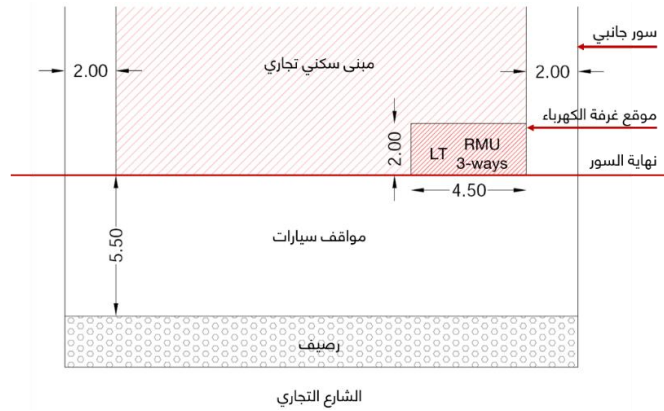
شكل رقم (٤٢) يوضح موقع وأبعاد غرفة الكهرباء
