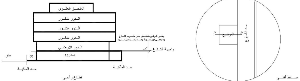
شكل رقم (١٤٣) دور التسوية في حال المبنى السكني على شارع واحد أعلى الارض
