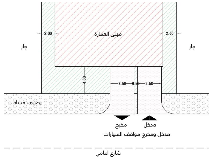
شكل رقم (٨٦) مدخل ومخرج مواقف السيارات بالعمارات السكنية
