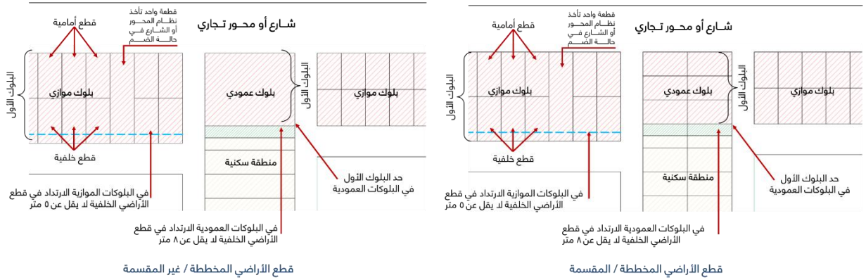
شكل رقم (٤٩) البلوكات العمودية والموازية
