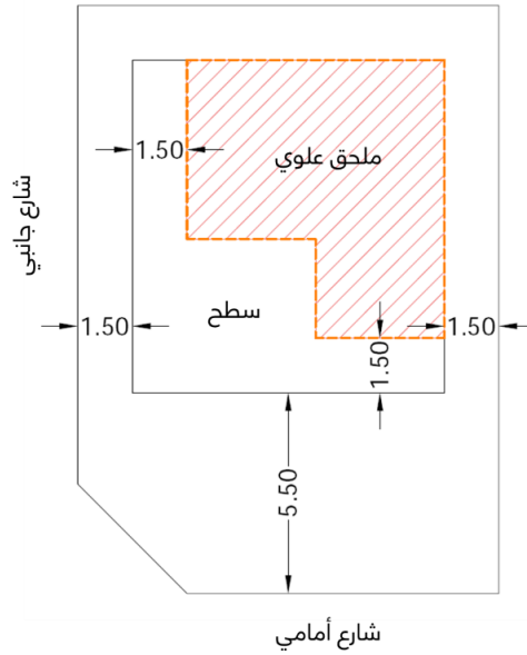
شكل رقم (٤٠) ارتدادات الملحق العلوي
