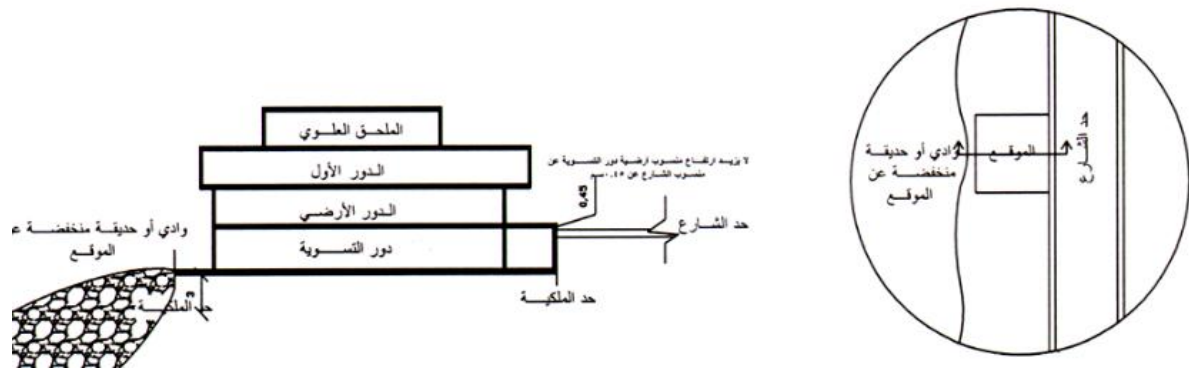
شكل رقم (١٤١) الناحية الخلفية أو الجانبية للموقع تطل على منطقة منخفضة عن منسوب الشارع بمقدار ٣م
