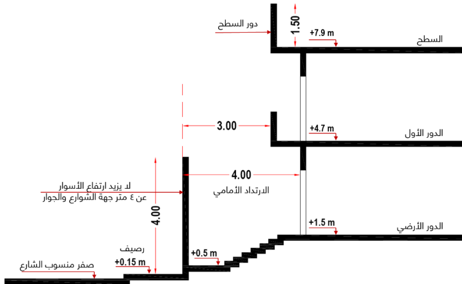
شكل رقم (٦٥) يوضح الحد الأقصى لارتفاع الأسوار بمباني الفيلات السكنية
