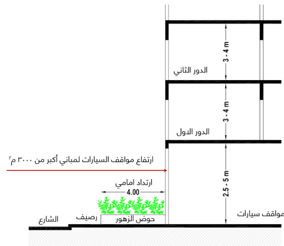
شكل رقم (٨٥) ارتفاع دور مواقف السيارات للمساحات أكبر من ٣٠٠٠ م ٢
