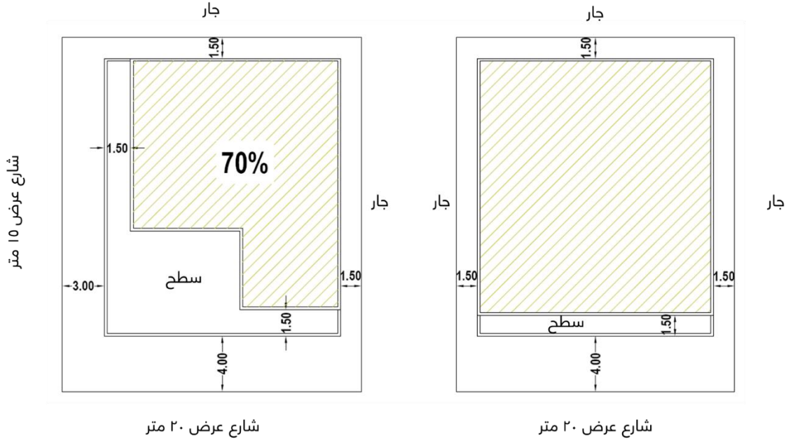
شكل رقم (٥٣) ارتداد الملحق العلوي عن حد الدور الذي بأسفله
