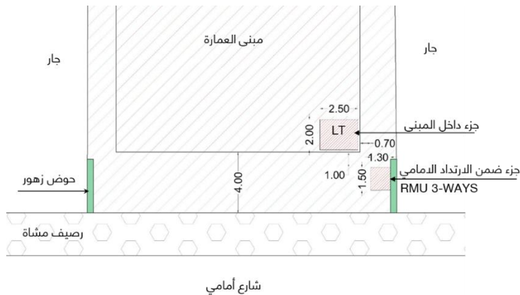
شكل رقم (٩٣) البديل الثالث موقع وأبعاد غرفة الكهرباء ضمن كتلة المبنى في المشاريع القائمة
