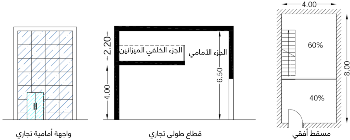
شكل رقم (٣٩) طابق الميزانين (الدور المسروق) في المحلات التجارية
