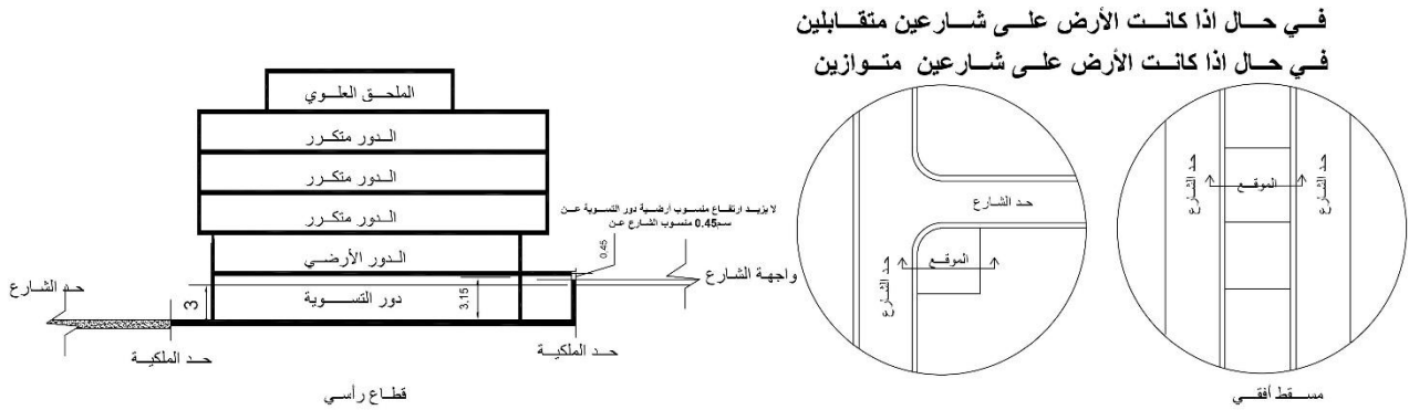
شكل رقم (١٤٢) دور التسوية في حال المبنى السكني على شارعين متقابلين او على شارعين متوازيين
