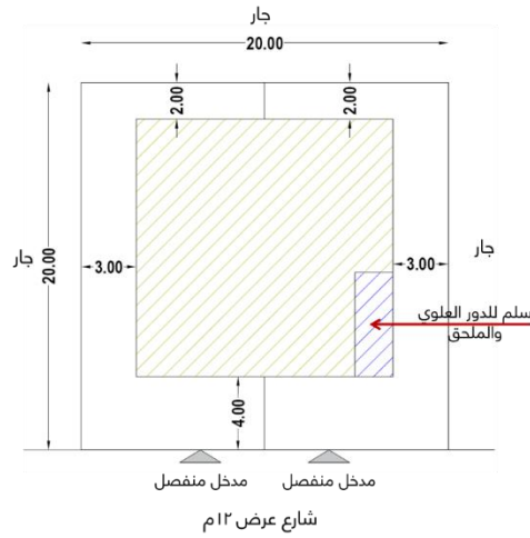
شكل رقم (٥٩) نموذج يوضح مداخل لوحدين سكنيتين (دور أرضي ودور علوي)
