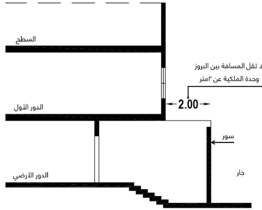
شكل رقم (٧٢) يوضح الحد الأدنى للبروز بالفيلات السكنية جهة الجوار
