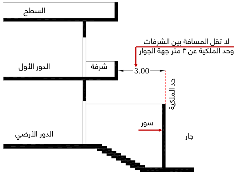
شكل رقم (٦٣) الحد الأدنى للارتداد جهة الجوار بالفيلات السكنية في حالة وجود شرفات
