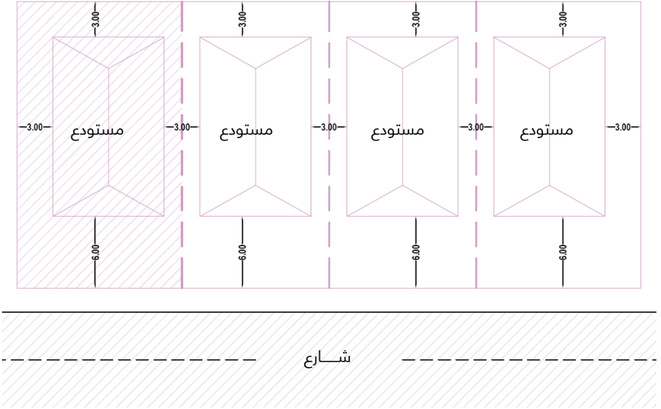
شكل رقم (٩٩) المستودعات متوسطة الخطورة الواقعة ضمن المناطق المخصصة للمستودعات أو المناطق الصناعية
