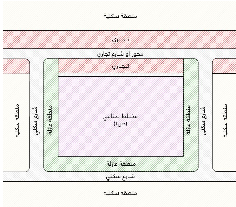
شكل رقم (٩٧) عزل المناطق الصناعية (ص١) عن المحاور أو الشوارع التجارية والمناطق السكنية
