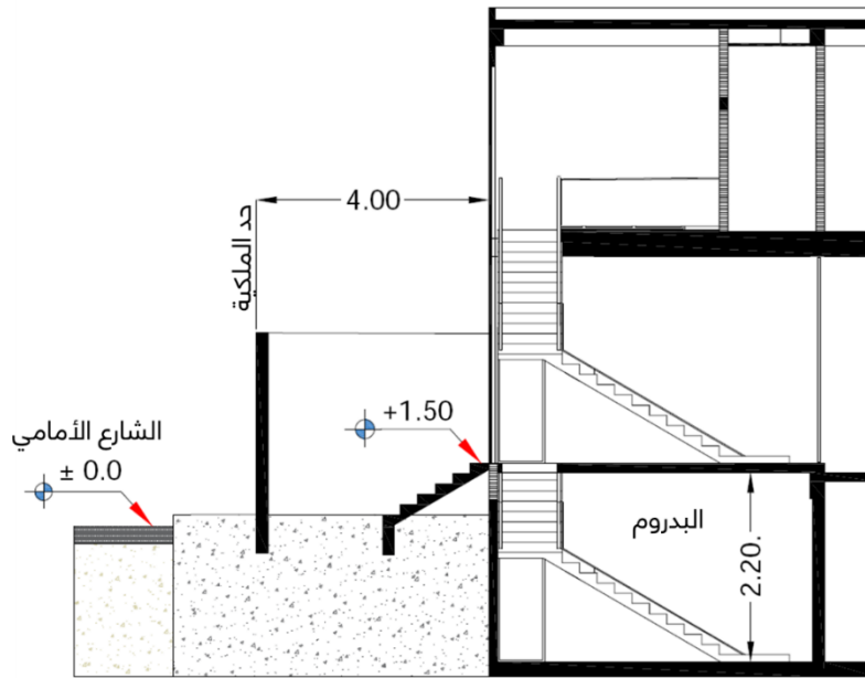
شكل رقم (٣٨) طابق البدروم (القبو)
