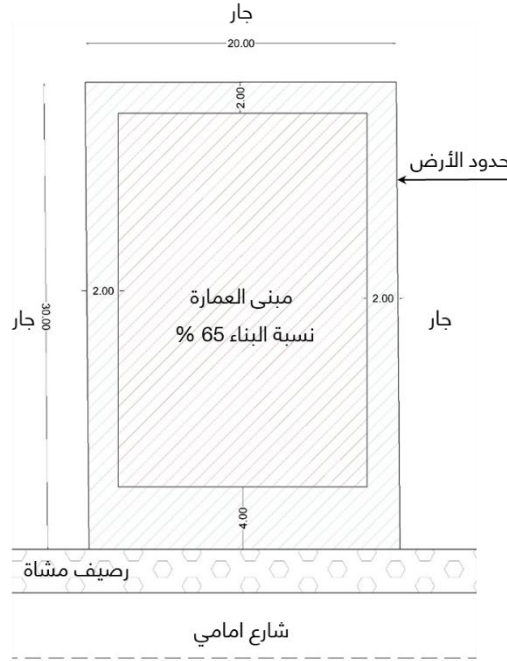
شكل رقم (٧٣) يوضح نسبة البناء بمناطق العمارات السكنية
