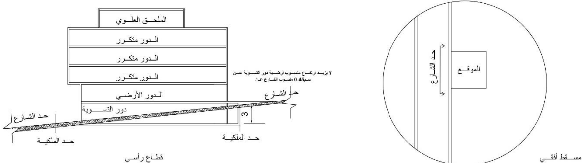
شكل رقم (١٤٤) دور التسوية في حال المبنى السكني على شارع واحد به ميل
