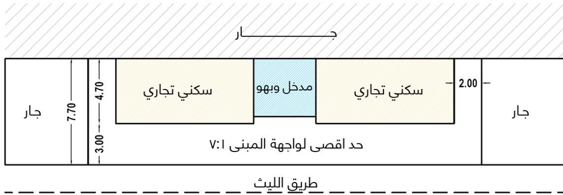
شكل رقم (٢٠) طريق الليث في حال الجار الخلفي مبنى
