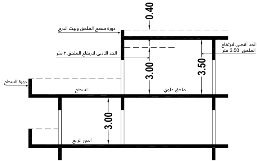
شكل رقم (٨٩) ارتفاع الملحق بمباني العمارات
