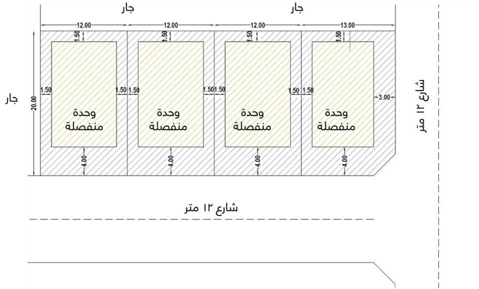
شكل رقم (٥٧) الحد الأدنى لعرض قطعة الأرض للفيلات متعددة الوحدات (المنفصلة)
