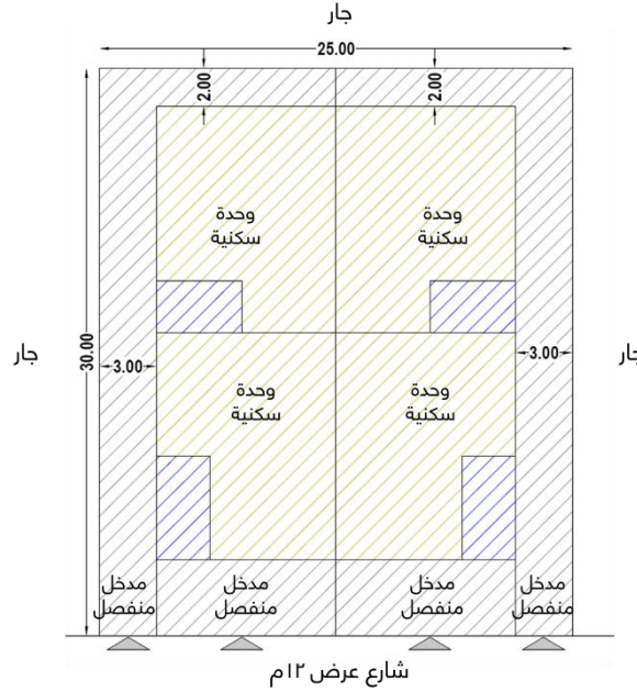
شكل رقم (١١) نموذج يوضح مداخل لأربع وحدات سكنية
