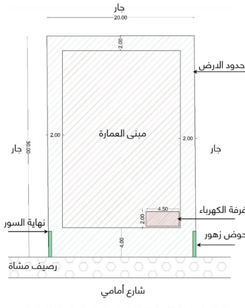
شكل رقم (٩١) البديل الثاني موقع وأبعاد غرفة الكهرباء بالعمارات السكنية الجديدة
