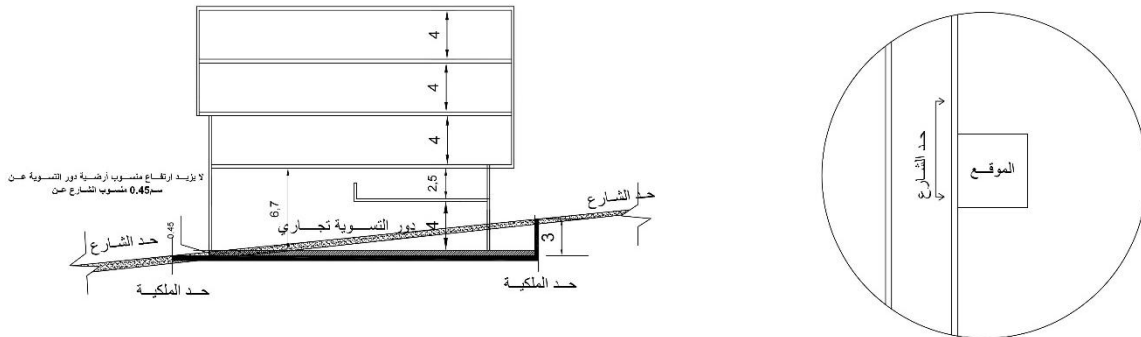
شكل رقم (١٤٦) دور التسوية في حال المبنى التجاري على شارع واحد به ميل
