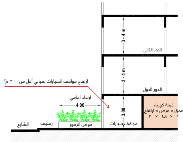
شكل رقم (٨٤) ارتفاع دور مواقف السيارات في حال وجود غرفة كهرباء
