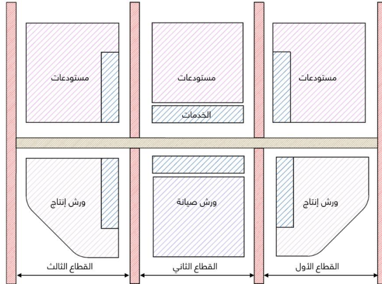
شكل رقم (٩٦) الدمج ما بين المستودعات والورش المهنية ضمن مخطط تقسيمي واحد
