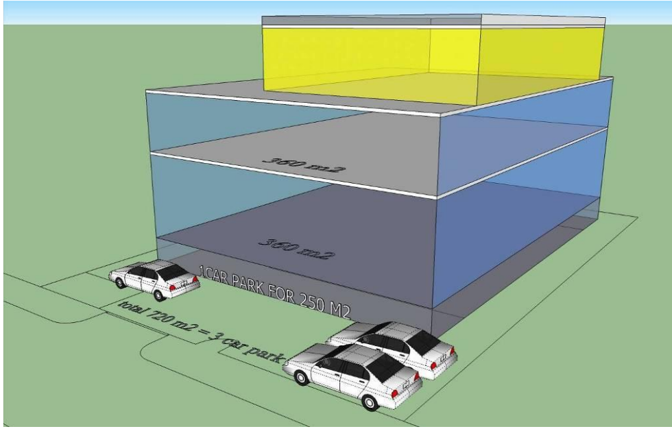
شكل رقم (٦٧) يوضح توفير مواقف السيارات المطلوبة داخل حدود الأرض وداخل السور
