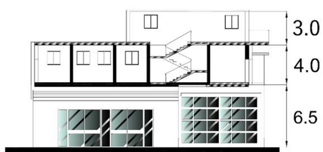
شكل رقم (٣٧) ارتفاع الطابق الأرضي مع طابق الميزانين
