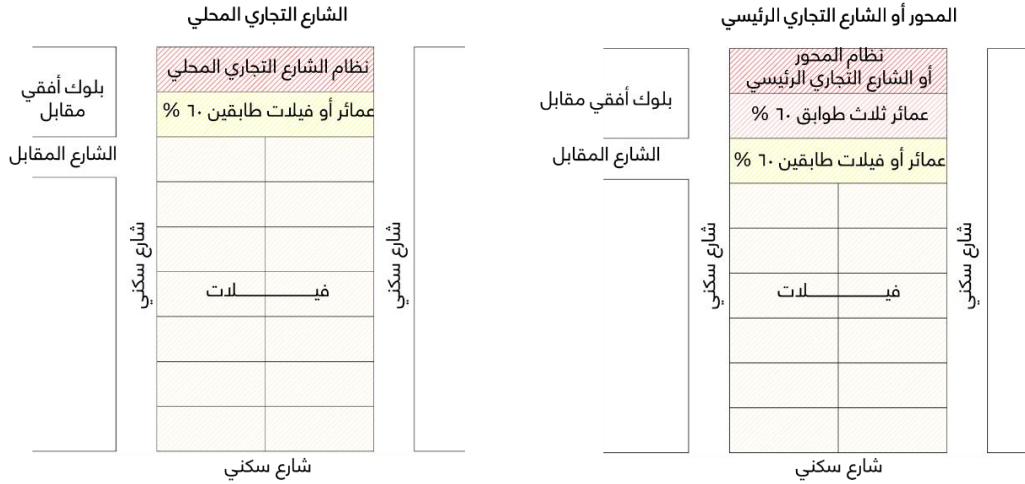
شكل رقم (٥١) نظام البناء للقطع الخلفية للبلوكات العمودية بمناطق الفيلات
