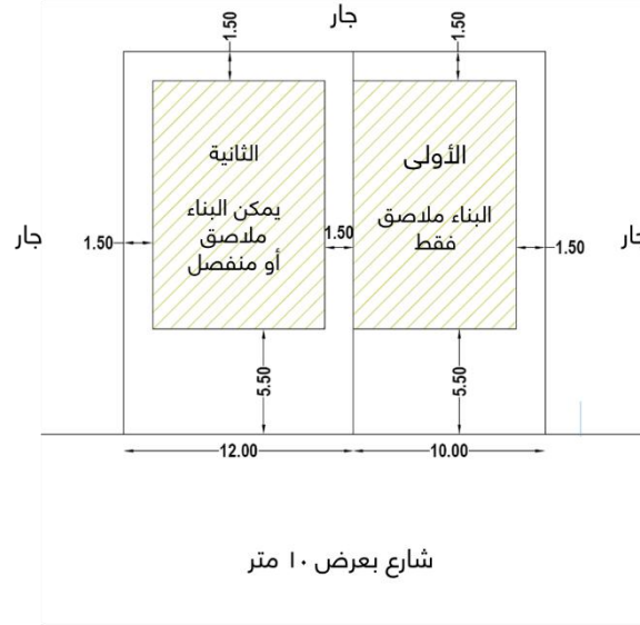
شكل رقم (٥٨) تجزئة الأرض إلى قطعتين أحدهما بواجهة ١٠م والأخرى ١٢م على الشارع
