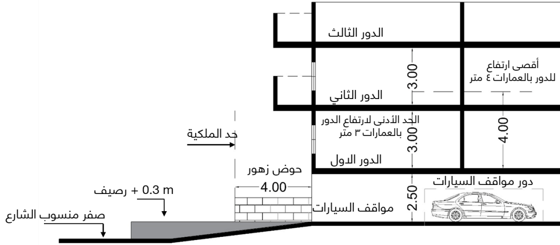
شكل رقم (٨١) ارتفاع دور مواقف السيارات للمساحات اكبر من ٣٠٠ م ٢
