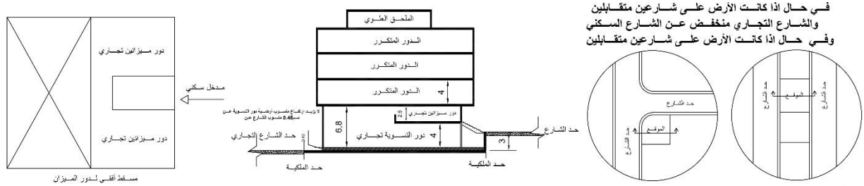
شكل رقم (١٤٧) دور التسوية في حال المبنى التجاري على شارعين متقابلين او على شارعين متوازيين (تجاري فقط)
