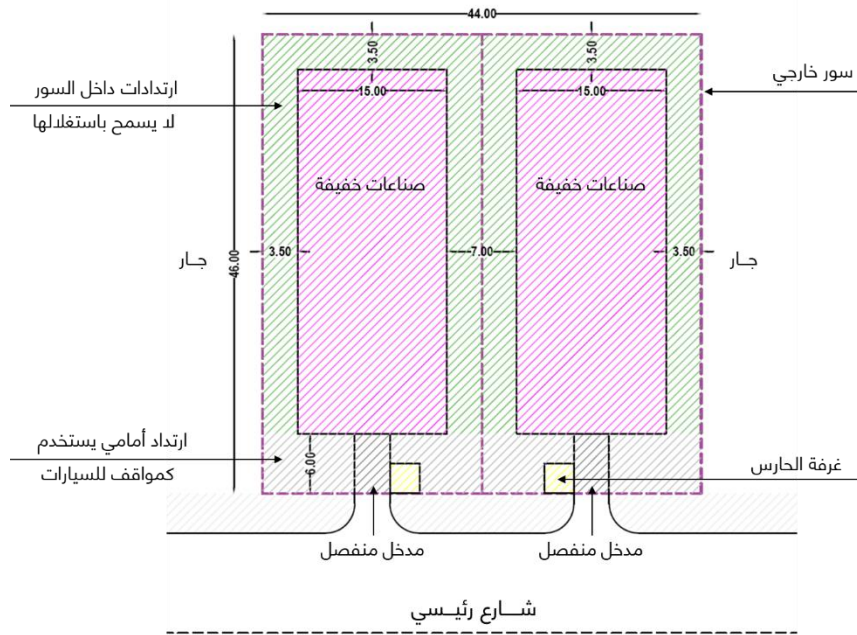
شكل رقم (١٠١) التعدد بالصناعات الخفيفة ضمن المناطق الصناعية (ص١)
